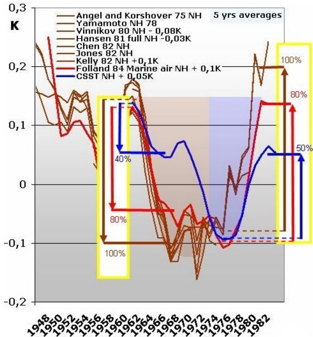
Abbildung 4: In dieser Illustration konnten wir bestätigen, dass sich die Lufttemperaturwerte an Land am schnellsten ändern („100%“), danach folgen die Lufttemperaturen über dem Wasser („80%“) und schließlich die SST, die das neue Temperaturniveau erreichen. Wieder sieht es so aus, dass sich nach einer bestimmten Zeit die Temperaturwerte von Festland und Ozean angleichen. Dies scheint sich innerhalb weniger Jahre abzuspielen, vor allem, wenn eine generelle Erwärmung bzw. Abkühlung unterbrochen wird oder sich umkehrt.
