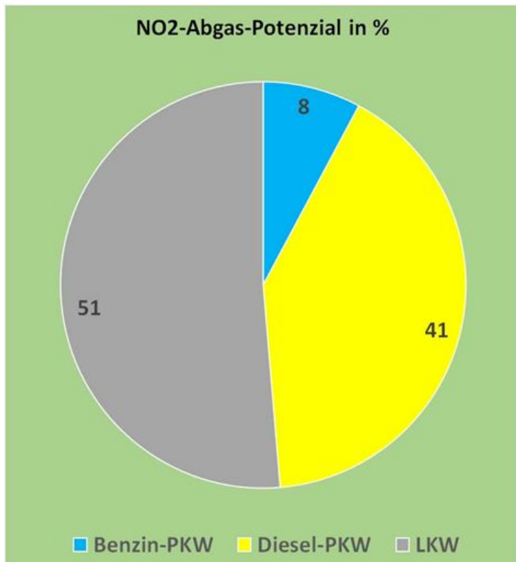
Bild 9. Das tatsächliche NO 2 -Immissionspotenzial des Abgases der verschiedenen Fahrzeugkategorien unter Berücksichtigung der Umwandlung von NO in NO 2 , berechnet auf Basis der Daten der Bilder 2 und 3
