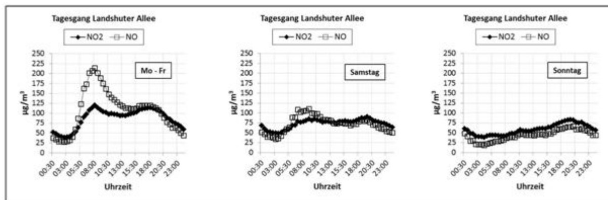
Bild 8. Mittlere Tagesgänge von \text{NO} und \text{NO}_2 am Münchner Brennpunkt Landshuter Allee an Wochentagen sowie an Samstagen und Sonntagen (Grafik: [BLFU])
