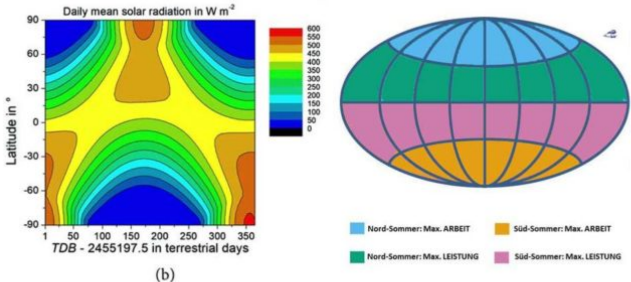
Abbildung 5: Zum Unterschied zwischen Leistung und Arbeit der solaren Einstrahlung. Links: Gemittelte 24h-tagesdurchschnittlich zurückgerechnete Strahlungsleistung der Sonne in Abhängigkeit von der Jahreszeit und der geographischen Breite über ein Jahr (Abbildung 22 b aus Kramm et al. (2017) : ... (b) solar radiation reaching the Earth's surface; ... as predicted for one year starting with TDB=2,455,197.5 (January 1, 2010, 00:00 UT1) – Creative Commons License CC BY 4.0). Rechts: Die maximale spezifische solare (Strahlungs-)LEISTUNG (~S-B-Temperaturäquivalent) und die maximale solare ARBEIT (Arbeit=Leistung x Zeit über die örtliche Tageslänge) im jeweiligen Sommerhalbjahr auf der Nord- und Südhalbkugel (nicht flächengetreu – weitere Erläuterungen sind hier zu finden)
