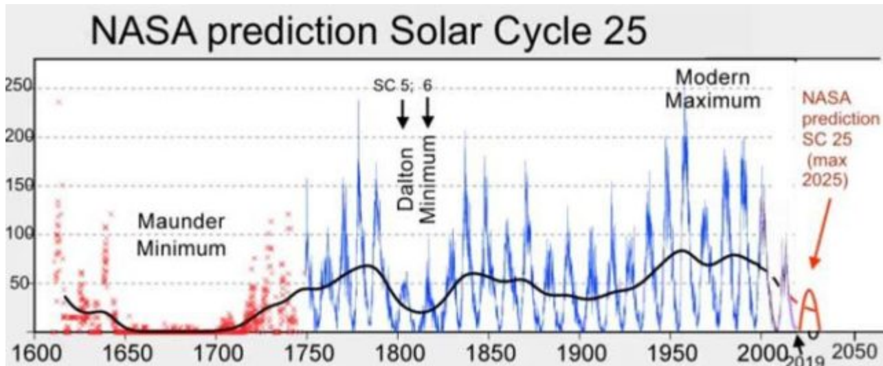
Abbildung 9: Die Vorhersage der NASA für den Sonnenzyklus 25 zeigt, dass er der schwächste der letzten 200 Jahre sein wird. (Abbildung aus einem EIKE-Artikel)
