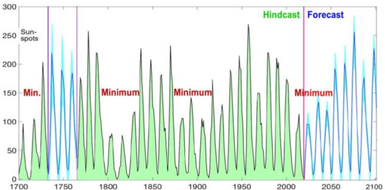
Abbildung 8: “The Sun may be quiet for half a century” aus der Presseerklärung von Velasco Herrera et al. (2021)
