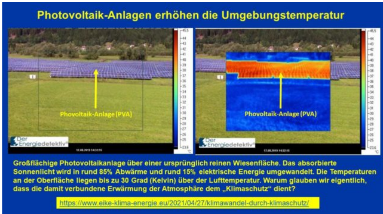
Abbildung 1: Solaranlage über einer Grünfläche. Das Wärmebild (rechts) macht die Emission von Wärme durch die Photovoltaik-Anlage deutlich
