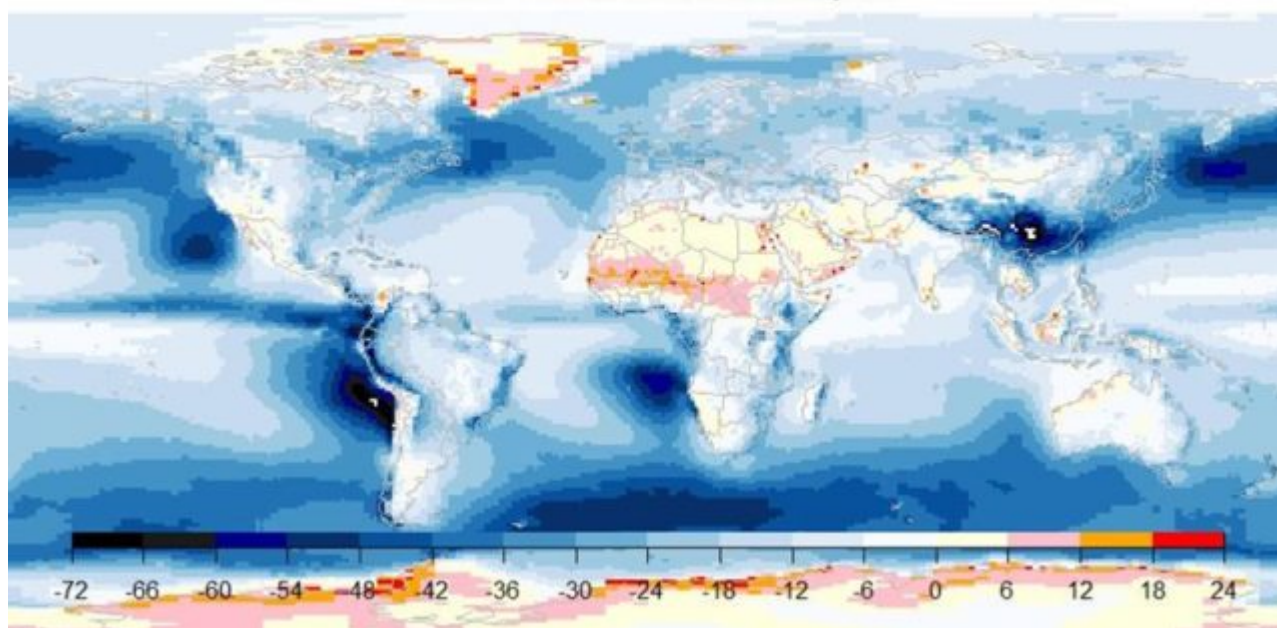
Abbildung 1. CRE in \text{W/m}^2 . Negative Werte (schwarz, grau und blau) bedeuten Abkühlung. Daten von https://ceres.larc.nasa.gov/data/
