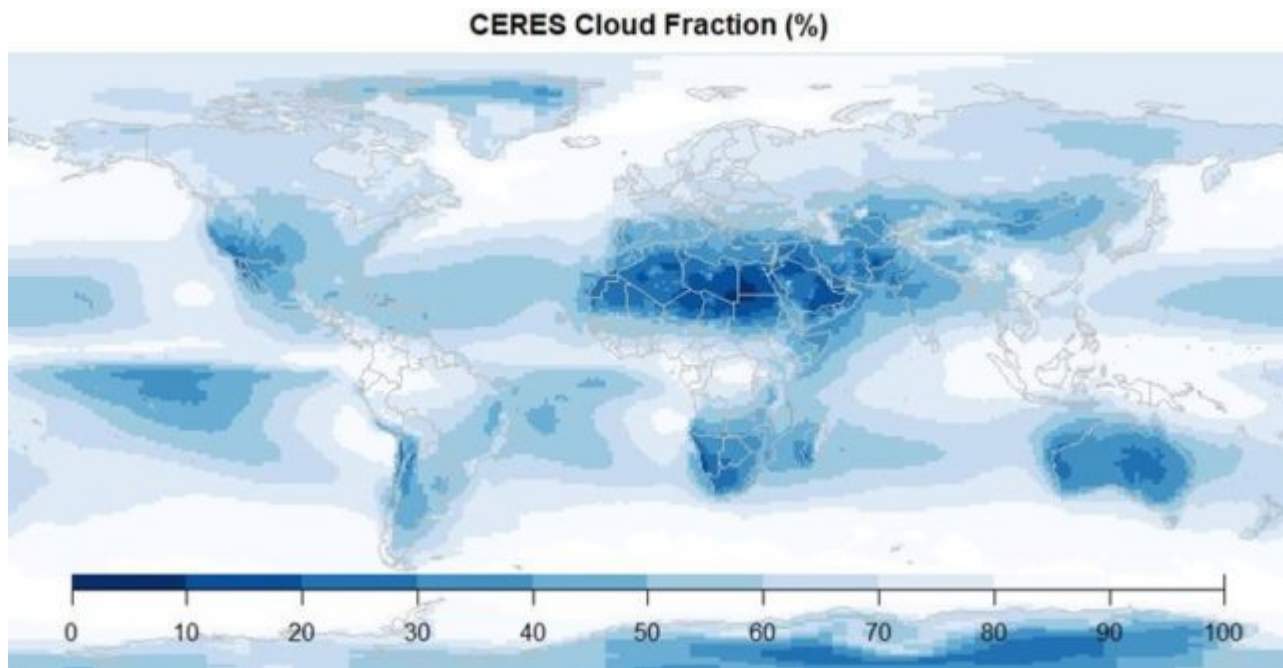
Abbildung 2. CERES-Wolkenanteil in Prozent. Dunklere Farben bedeuten weniger Bewölkung, hellere Farben bedeuten mehr Wolken.
