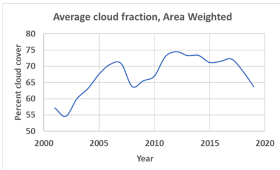
Abbildung 5. CERES Durchschnittlicher monatlicher Wolkenanteil, Variable cldarea_total_daynight_mon .
