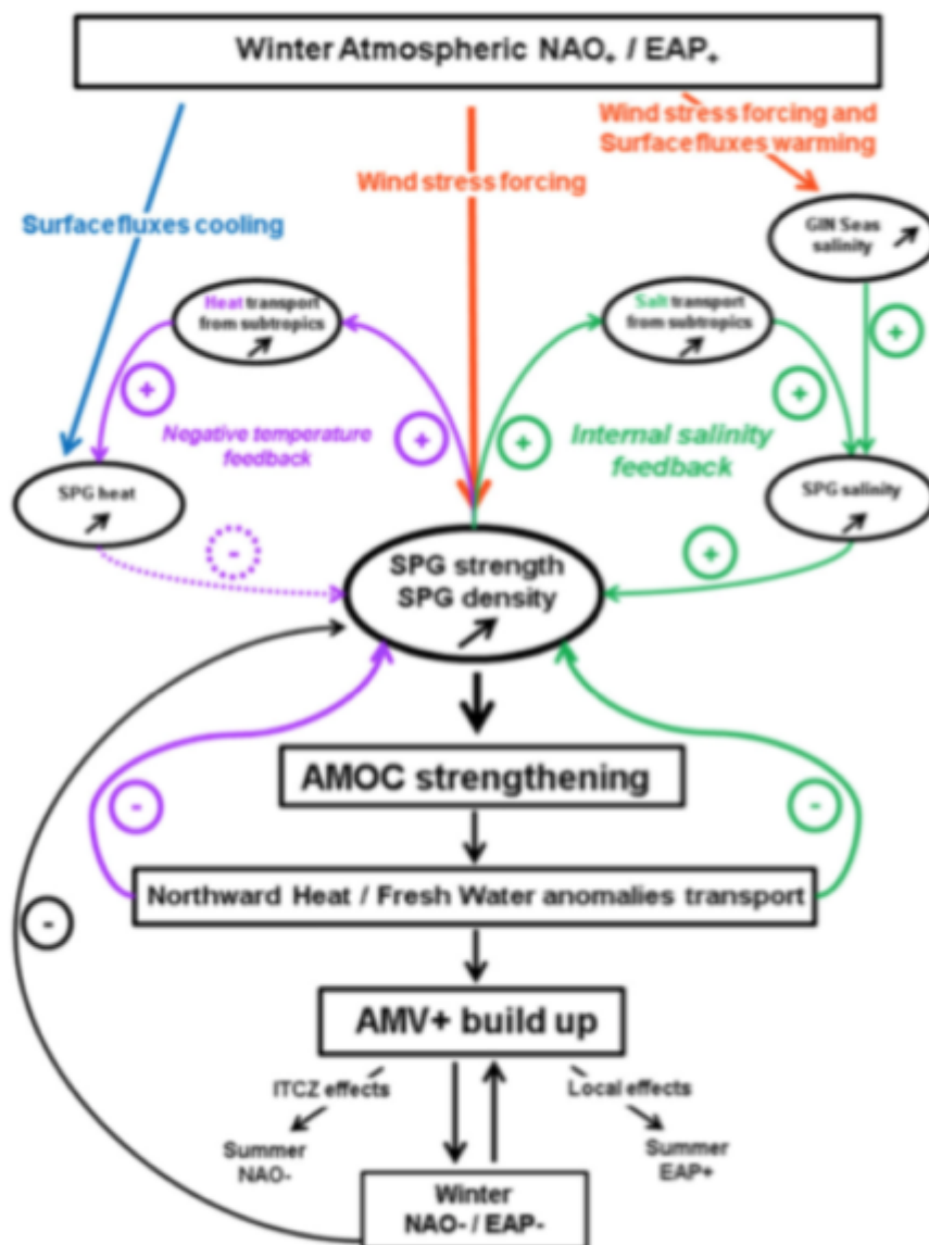
Abbildung 9.8: Schematisches Diagramm für ein Positiv-Ereignis von AMOC/AMV. Nach RuprichRobert und Cassou (2014)
