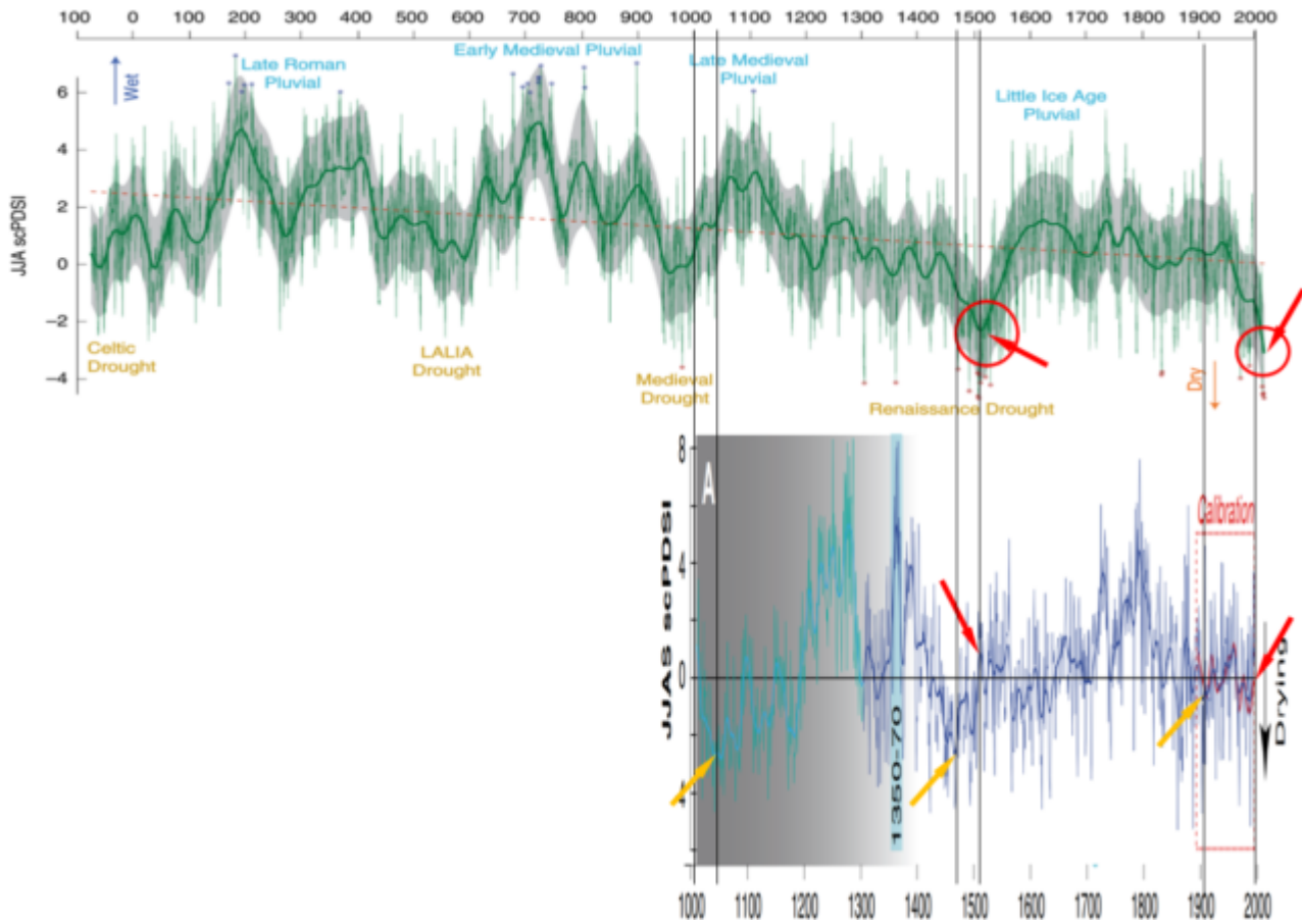
Bild 10 Zusammenstellung Büntgen 2020 [1] und Büntgen 2010 [4] im gleichen Maßstab. Grafik vom Autor erstellt Es ist allerdings nicht so, dass Herr Büntgen solches nicht bemerken würde. In den Supplements zur Studie gibt es dazu eine Gegenüberstellung:
