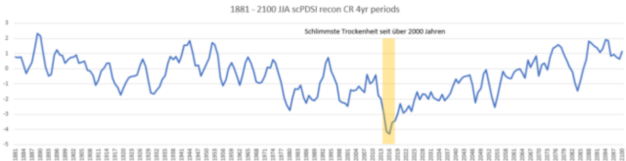
Bild 7 Sommervariabilität des Trockenheitsindexes von 1881 – 2100. Grafik vom Autor anhand der Daten [1] und Annahmen erstellt. Das widerspricht zwar etwas der Klimasimulation des DWD für Deutschland. Aber in diese sind die „Erkenntnisse“ der Studie sicher noch nicht eingearbeitet.
