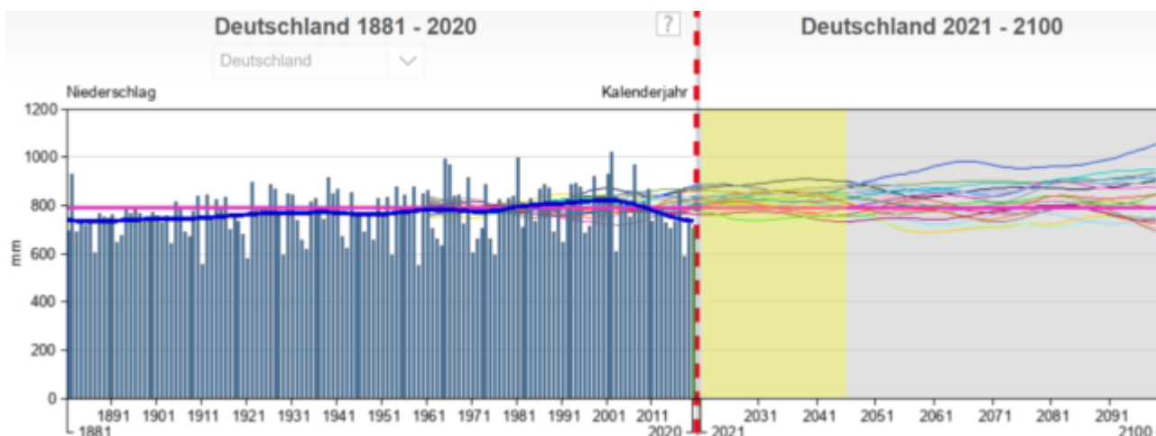
Bild 9 Deutschland, Jahresniederschlag von 1881 – 2100. Quelle: DWD-Datenviewer
