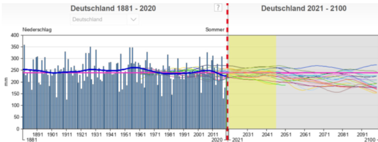
Bild 8 Deutschland, Sommerniederschlag von 1881 – 2100. Quelle: DWD-Datenviewer
