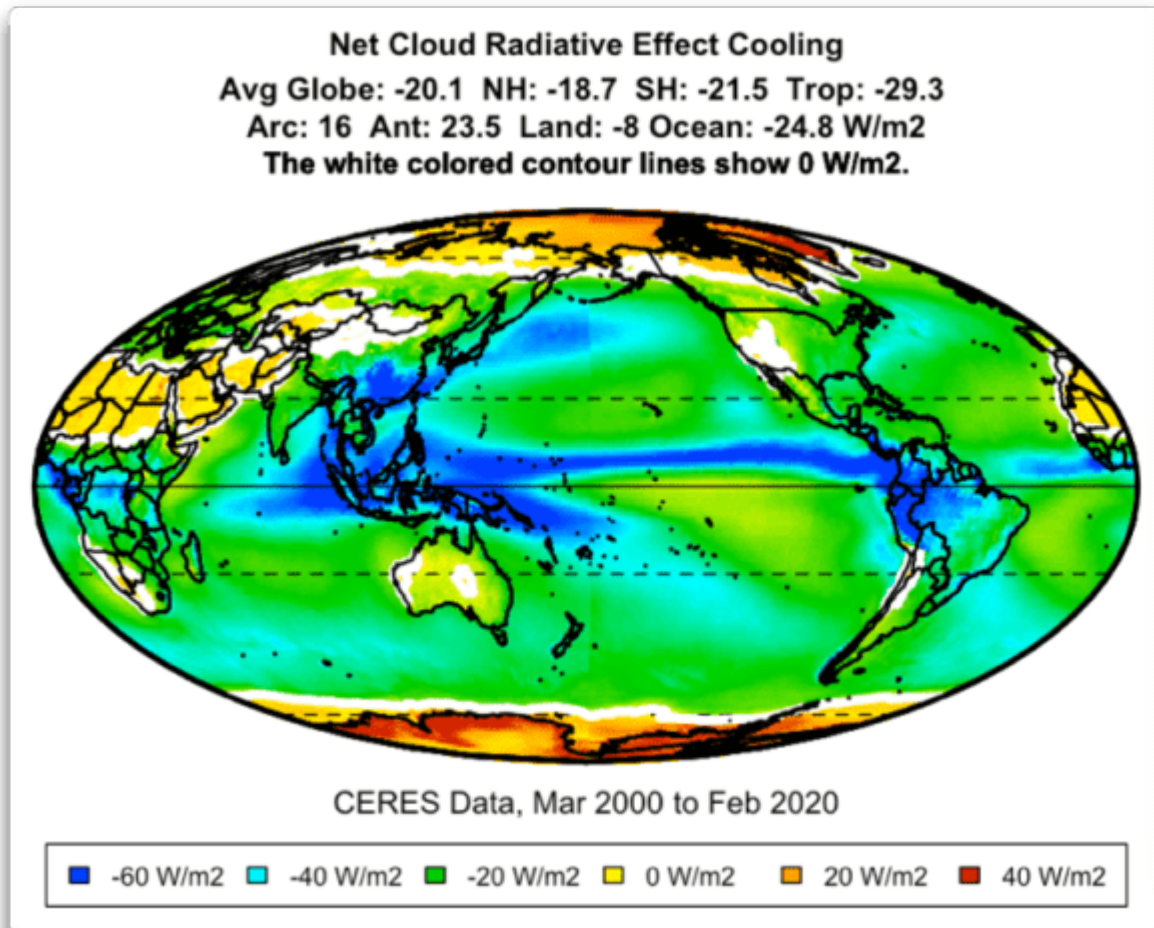
Abbildung 1. Netto-Wolkenstrahlungseffekt (LW-Erwärmung minus SW-Abkühlung)
