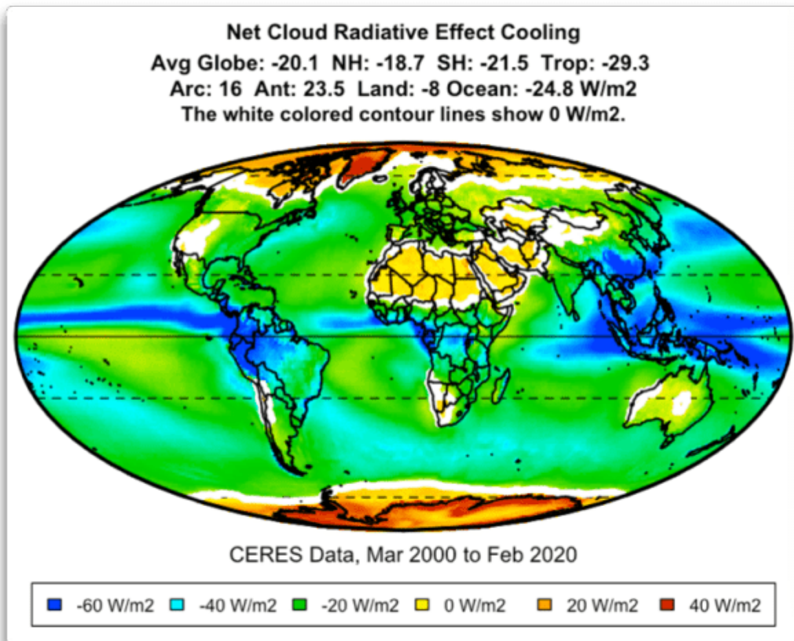
Abbildung 2. Wie in Abbildung 1, atlantische Seite. Netto-Strahlungseffekt der Wolken (LW-Erwärmung minus SW-Kühlung)
