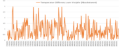
Station Berlin-Dahlem. Temperaturdifferenz zum Vorjahr (Absolutwerte) 1711 – 2019. Grafik vom Autor anhand der DWD-Daten erstellt
