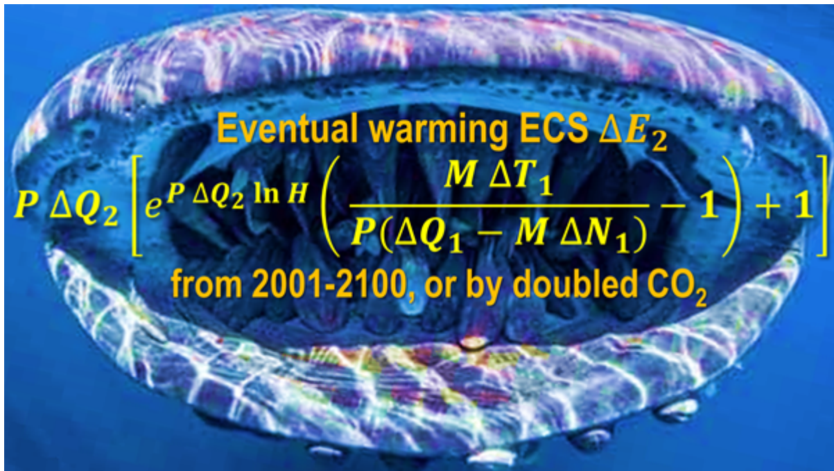
Abb. 5: Die Monster-ECS-Gleichung: einfacher, billiger, smarter als jedes Giganten-Klimamodell
