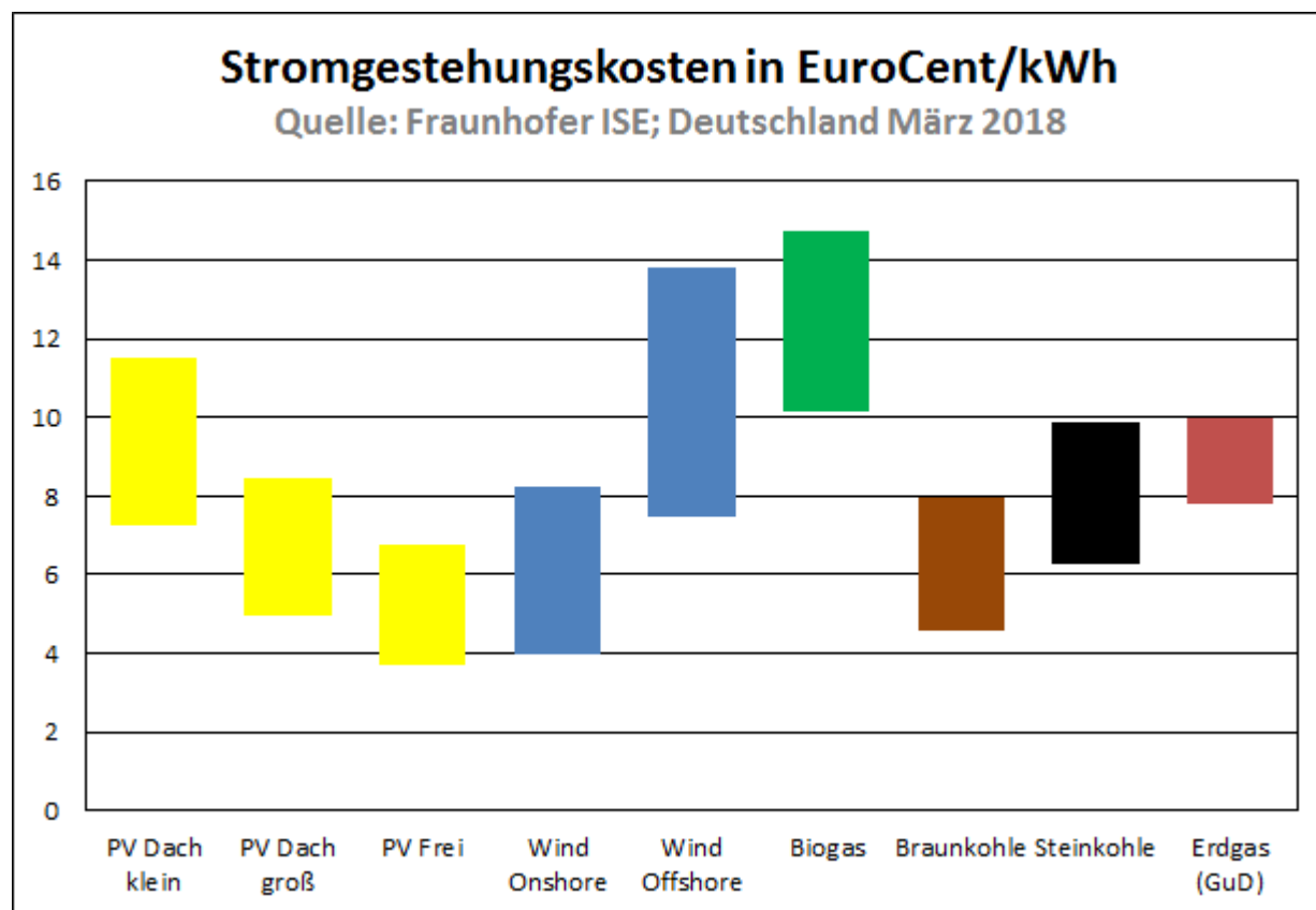
Stromgestehungskosten_Deutschland_2018_laut_Fraunhofer_ISE
