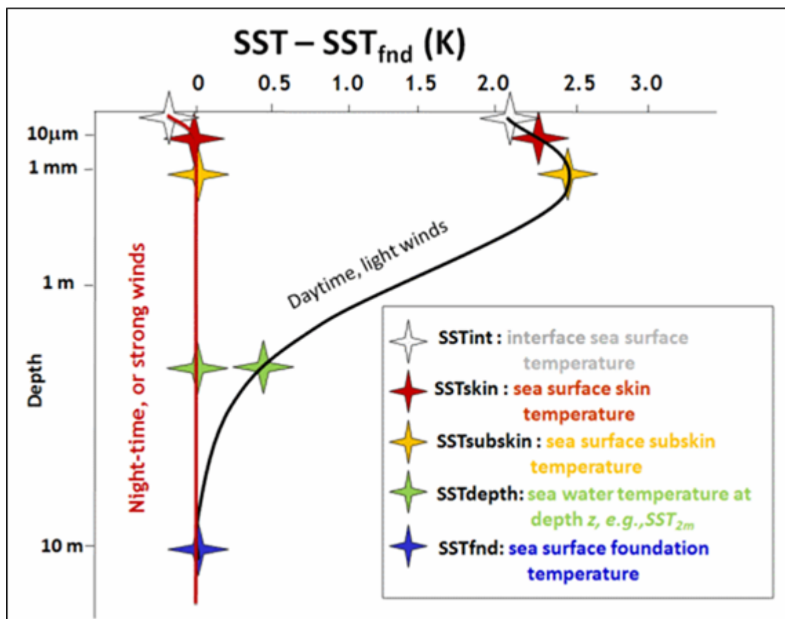
Abbildung 1. Das GHR SST-Diagramm der Temperatur an der Meeresoberfläche. Die Meeresbedingungen, insbesondere die Windgeschwindigkeit und die Tages- oder Nachtzeit, können einen Unterschied von 2,5 °C oder mehr im Temperaturgradienten von der Oberfläche zur Temperatur des Untergrunds (stabiler Teil der Mischschicht) ausmachen. Die Tiefe bis zum oberen Ende des
