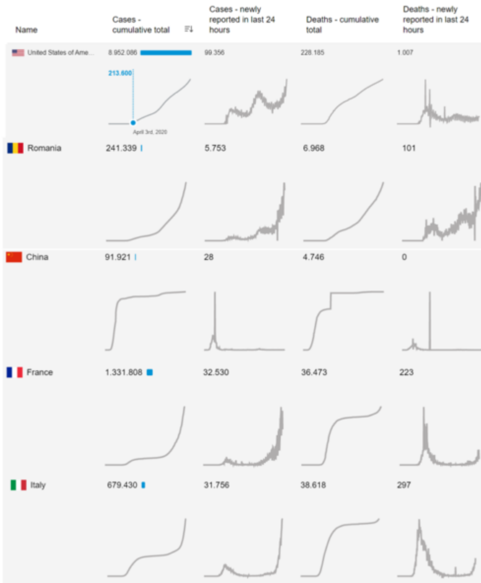
Bild 19 Corona-Verlaufsgrafiken einzelner Länder.
