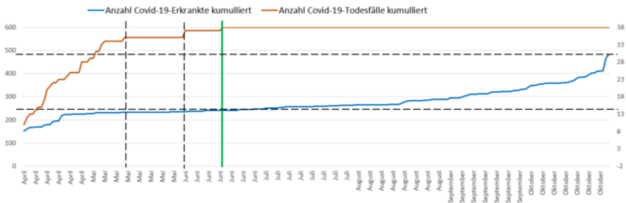
Bild 2 Coronadaten Fürth. Verlauf Covid-19-Erkrankte und Todesfälle. Grafik vom Autor erstellt. Datenquelle: corona-fallzahlen.landkreis-fuerth.de
