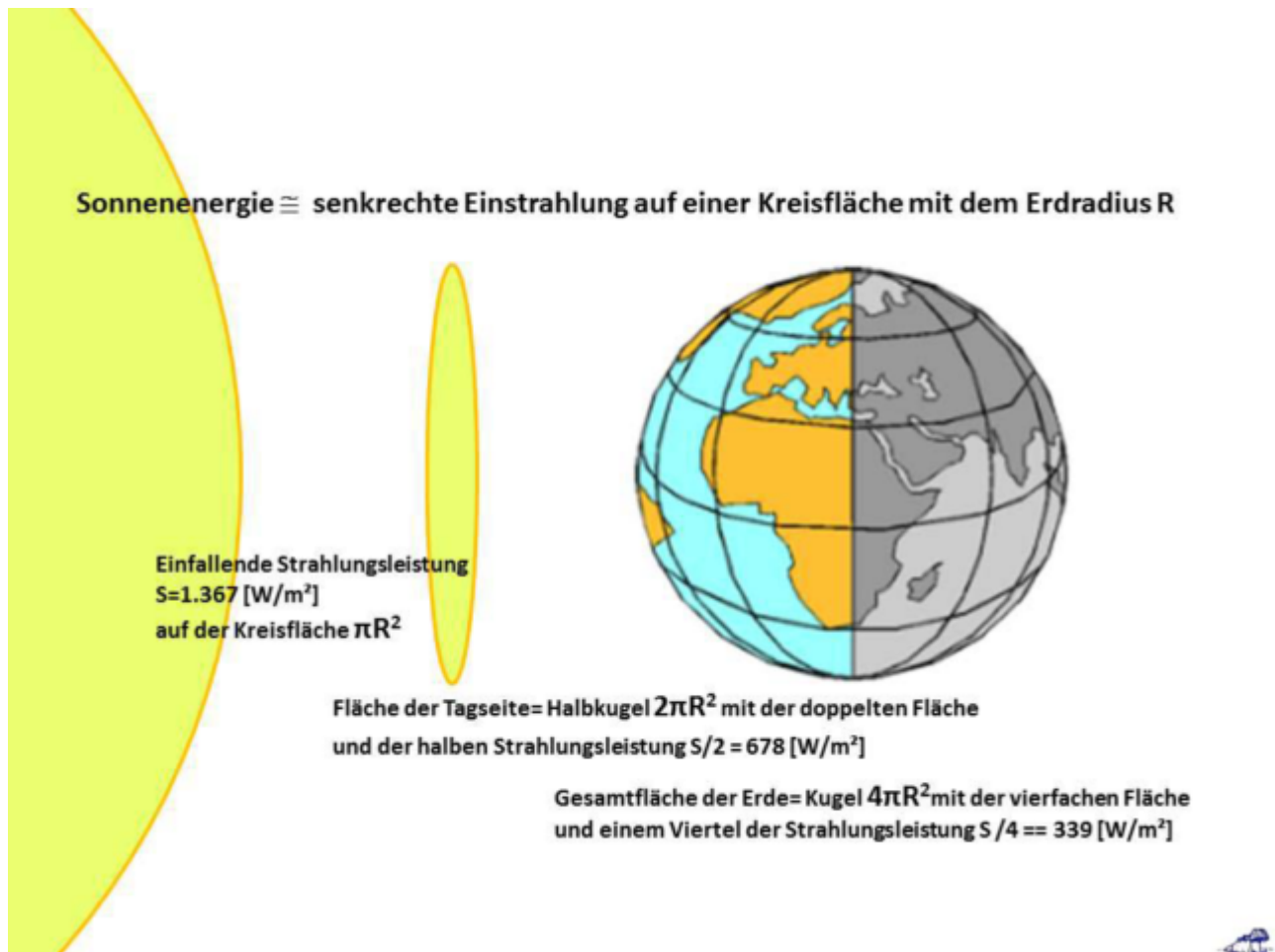
Abbildung: Das hemisphärische S-B-Modell für die Temperaturogenese auf unserer Erde
