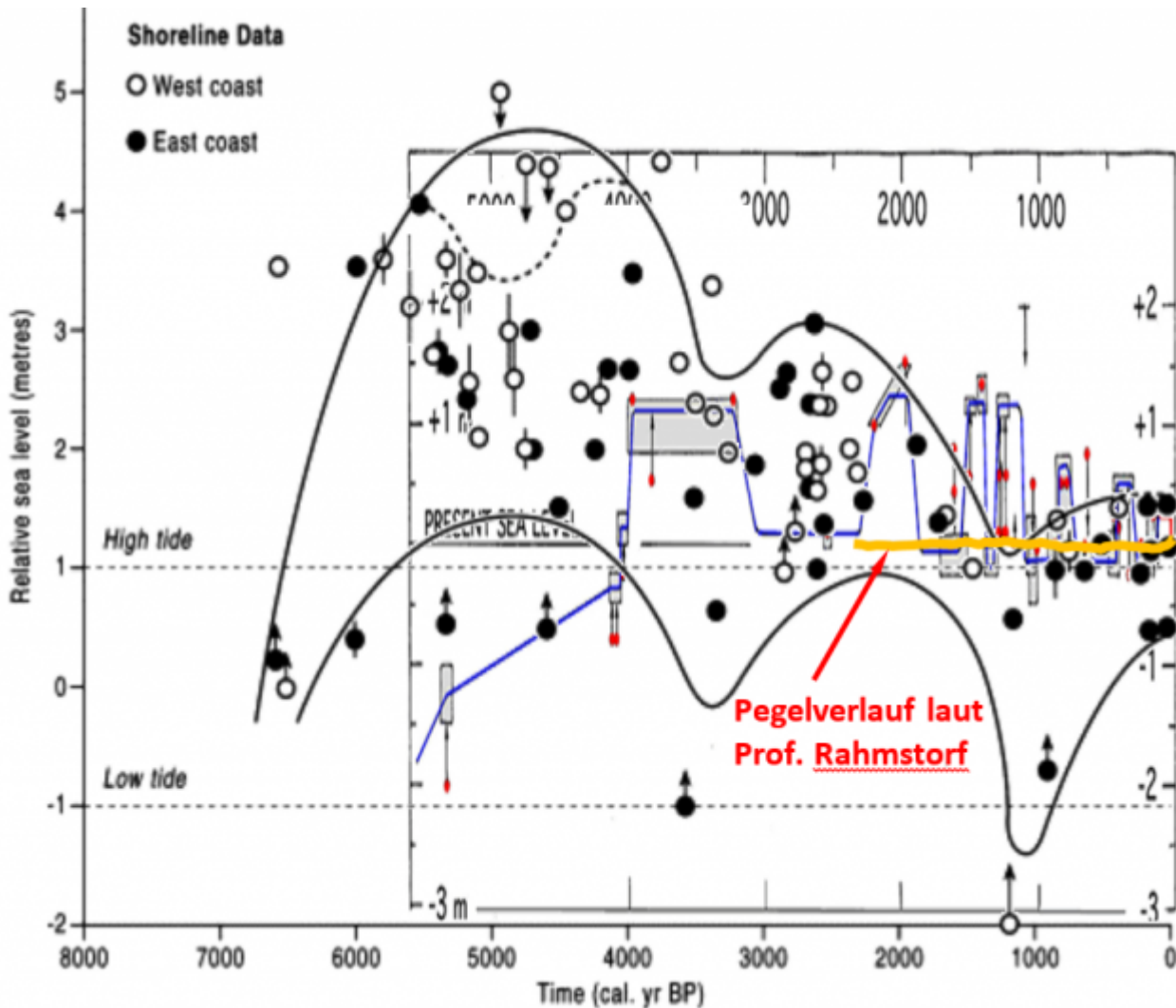
Bild 30 Rekonstruktionsversuch Pegelverlauf der letzten 3000 Jahre. Bilder 3; 7; 21 im gleichen Zeit- und Höhenmaßstab vom Autor übereinander kopiert. Hinweis: Die 0-Linien der Proxy-Y-Achsen sind versetzt. Die Pegelspannen aber im Maßstab
