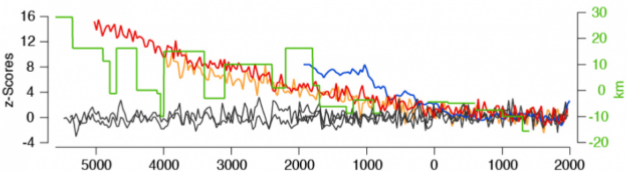
Bild 27 Temperaturtrend seit ca. 7000 Jahren in nördlichen Breitengraden. [8]
