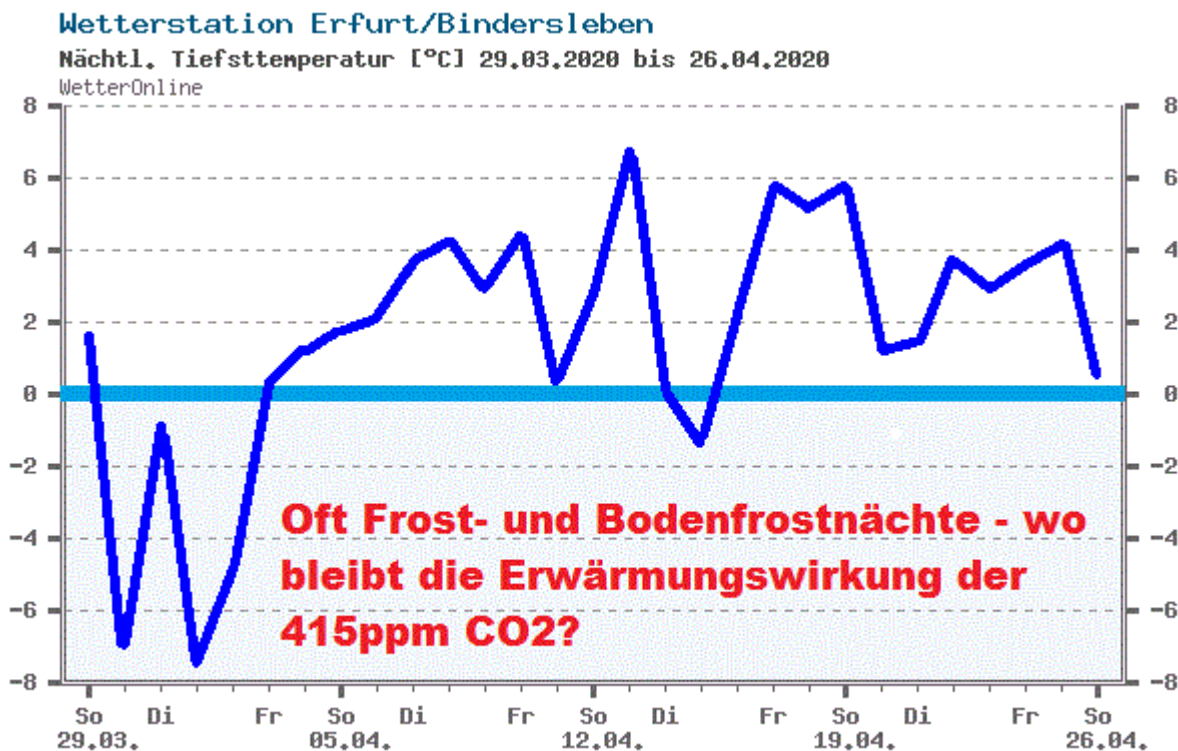
Abbildung 1: Verlauf der Tagesminima (°C) an der DWD-Station Erfurt/Weimar vom 29. März bis zum 26. April 2020. Antizyklonale Kaltfronten lenkten immer wieder trockene Nordluft nach Deutschland – und nur tagsüber wärmt eben die Sonne, das CO 2 aber niemals. So
