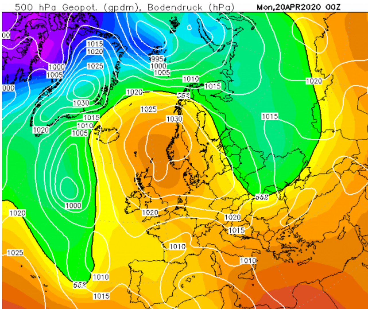
Abbildung 2: Wetterkarten-Ausschnitt vom 20. April 2020, 1 Uhr. Ein kräftiges Hochdruckgebiet über dem Nordmeer und Skandinavien lenkt trocken-kalte Festlandsluft aus Nordosten nach Deutschland. Dabei reichte hohes Geopotential (orange) von Nordafrika bis zum Nordmeer; entfernt erinnert seine Form an den griechischen Buchstaben Omega. Solche Lagen sind sehr stabil. Weil Deutschland meist knapp auf der Ostseite des „Omegas“ lag, herrschte zwar Hochdruckeinfluss vor, doch immer wieder konnte Kaltluft aus Norden „einsickern“. Quelle der Karte wetterzentrale.de ; Ausschnitt.
