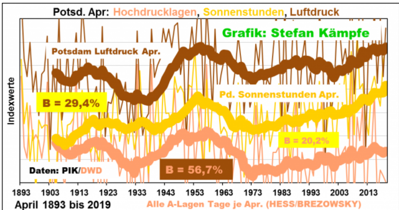
Abbildung 11: Der Luftdruck beeinflusste im April die Variabilität der
