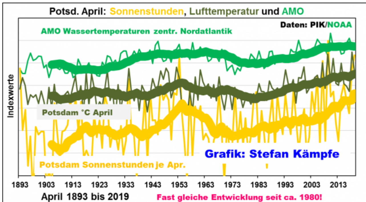
Abbildung 5: Fast Gleichklang zwischen der AMO, einem Index der Wassertemperatur im zentralen Nordatlantik, der Apriltemperaturen und der Sonnenscheindauer. Einer sehr sonnigen Mitte des 20. Jahrhunderts folgte eine Depression; aber nie seit Aufzeichnungsbeginn 1893 waren die Aprilmonate derart sonnig und warm, wie momentan. Der „Gleichklang“ legt einen Einfluss der AMO nahe. Zur Darstellung in einer Grafik mussten die sehr unterschiedlichen Größen in Indexwerte umgerechnet werden.
