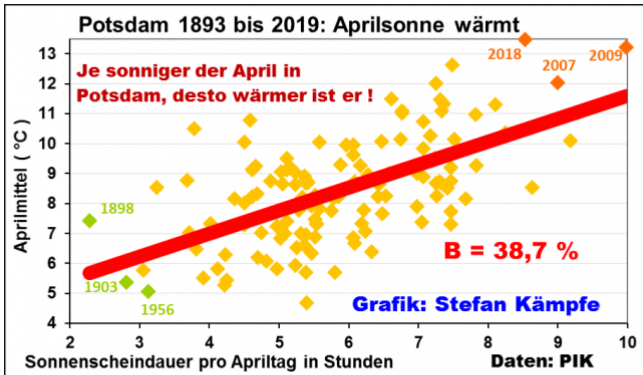
Abbildung 9: In Potsdam, wo seit 1893 auf dem Telegrafenberg gemessen wird, beeinflusste die Sonnenscheindauer die Variabilität der Apriltemperaturen zu mehr als einem Drittel, das ist wegen des hohen Stichprobenumfangs signifikant. Einige herausragend sonnig-warme und trüb-kalte Aprilmonate sind markiert. Der April 2020 wird ähnlich sonnig, aber wegen des vielen Nordwetters weniger warm als die Rekordmonate 2007, 2009 und 2018 ausfallen. Freilich haben auch andere Faktoren, wie die Strömungsrichtung, Einfluss auf die Apriltemperaturen.
