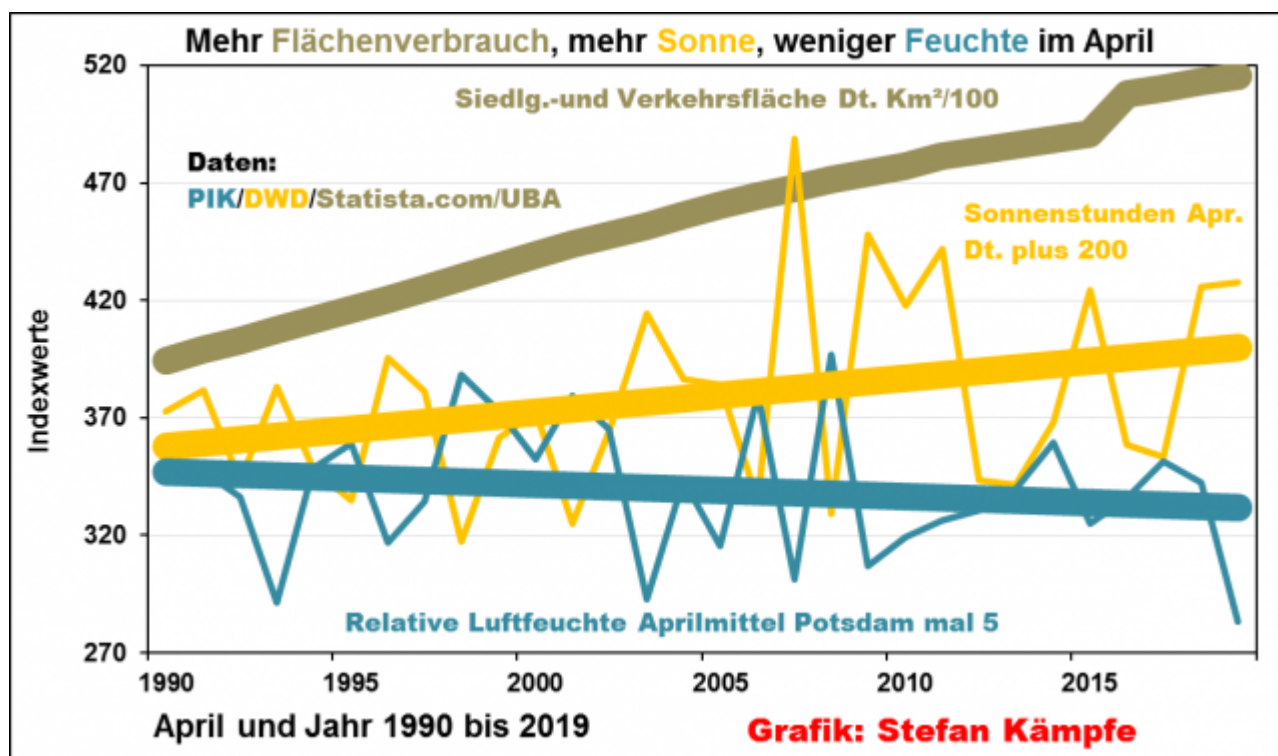
Abbildung 16: Die ständig wachsende Siedlungs- und Verkehrsfläche in Deutschland, von etwa 39.000Km 2 im Jahr 1990 auf etwa 51.500Km 2 im Jahre 2019, ging mit einer steigenden April-Sonnenscheindauer bei sinkender relativer Luftfeuchtigkeit einher. Zur Darstellung in einer Grafik mussten die sehr unterschiedlichen Größen in Indexwerte umgerechnet werden.
