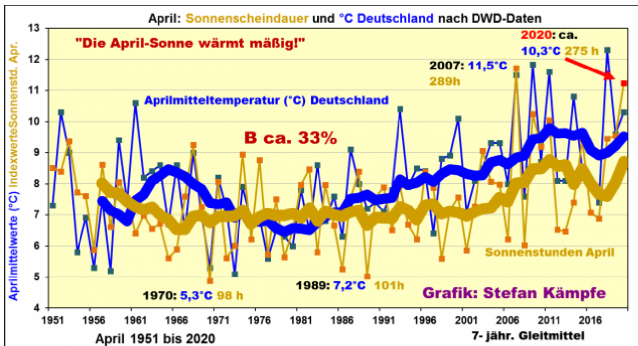
Abbildung 4: Eine merkliche Zunahme der Sonnenscheindauer ist eine wesentliche, aber nicht die alleinige Ursache für die steigenden April-Temperaturen; sie beeinflusste deren Variabilität aber zu immerhin einem Drittel. Eine weitere Ursache der April-Erwärmung ist eine Häufigkeitszunahme bestimmter Großwetterlagen. Werte für April 2020
