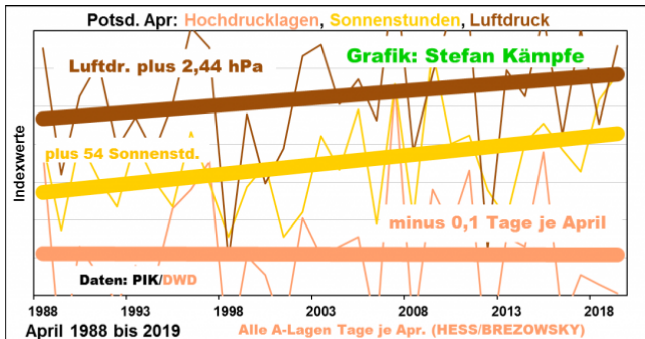
Abbildung 12: Seit 1988 blieb die Anzahl der antizyklonalen Großwetterlagen im April nahezu unverändert – aber Luftdruck und Sonnenscheindauer stiegen merklich an. Zur Darstellung in einer Grafik mussten die sehr unterschiedlichen Größen in Indexwerte umgerechnet werden.
