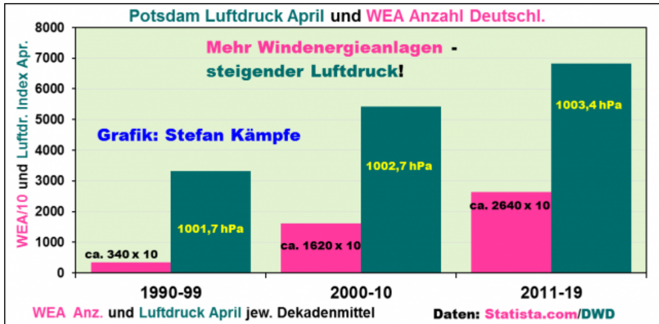
Abbildung 13: Mit dem dekadeweisen Ausbau der Windenergie stiegen auch die Luftdruckwerte im April merklich. Der Luftdruck musste zur besseren Darstellung beider Größen in einer Grafik in Indexwerte umgerechnet werden; die wahren, in Potsdam nicht auf NN reduzierten Werte siehe in den grünen Säulen.
