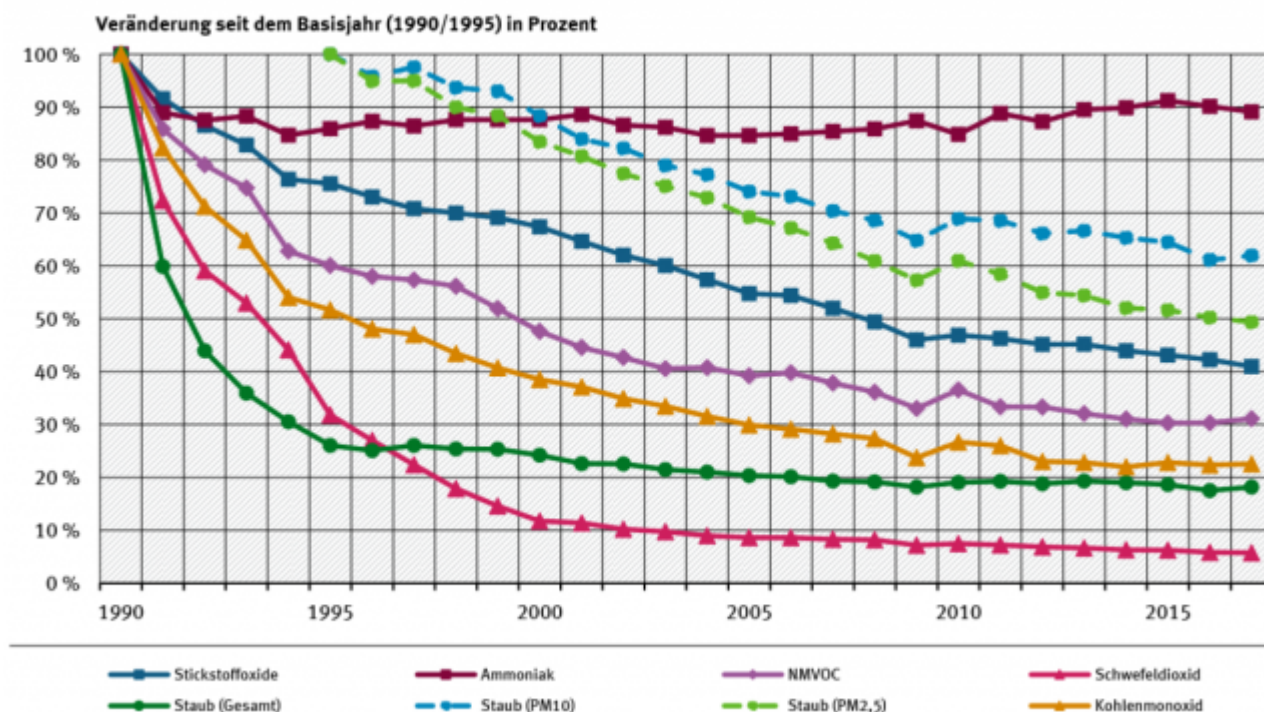
Bild 8.2 Beispiel Deutschland: Relative Veränderungen von Luftschadstoffen in Deutschland über die Jahre. Quelle: UBA
