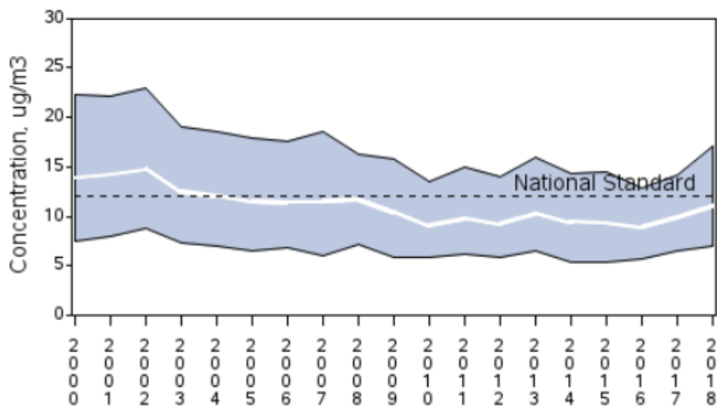
Bild 8.1 USA: Beispielhafter Verlauf und Streuung von Feinstaub im Studienzeitraum (2000 ... 2016)
