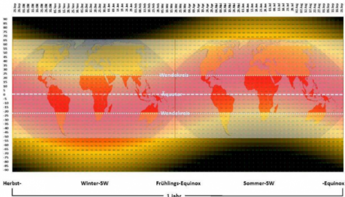
Abbildung: Tentative Gegenüberstellung der Beleuchtungsklimazonen mit dem Jahresverlauf der maximalen solaren Strahlungsleistung im Sommerhalbjahr (Südsommer linke Hälfte und Nordsommer rechte Hälfte) Overlays rechts und links: Die Beleuchtungsklimazonen der Erde: von oben/unten zur Mitte: Polarzonen, Mittelbreiten, Tropenzone (Quelle: Wikipedia , Autor: Fährtenleser , Lizenz: GNU Free Documentation License ) Darunter: Das örtliche Maximum der breitenabhängigen temperaturwirksamen spezifischen Strahlungsleistung der Sonne für die gesamte Erde über ein volles Jahr von Herbstäquinoktium zu Herbstäquinoktium
