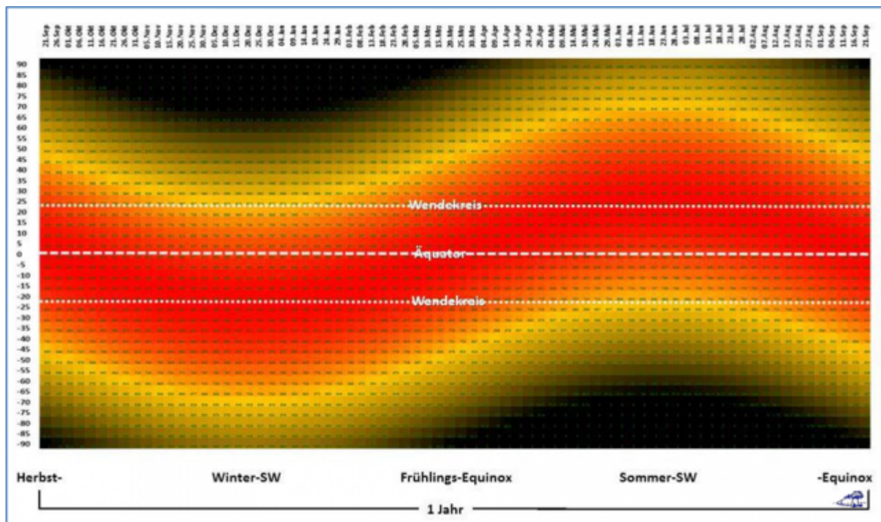
Abbildung: Das örtliche Maximum der breitenabhängigen temperaturwirksamen spezifischen Strahlungsleistung der Sonne für die
