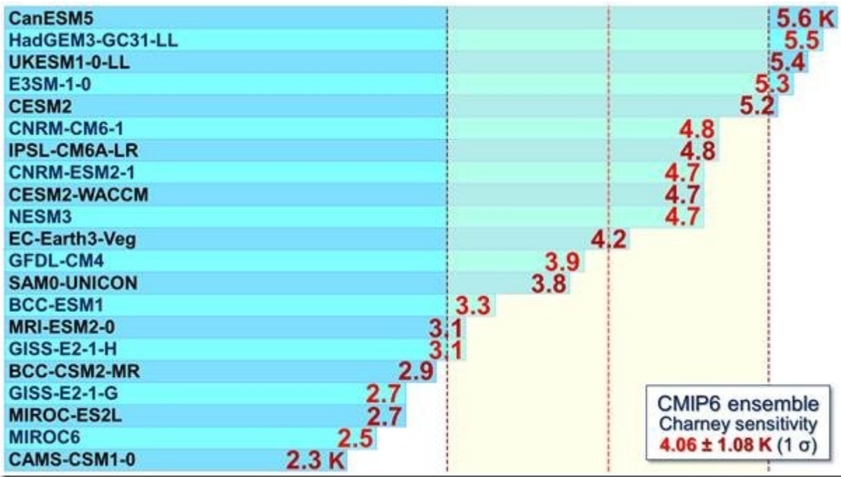
Abbildung 5: Projektionen der Charney-Sensitivität in 21 Modellen des CMIP5-Ensembles
