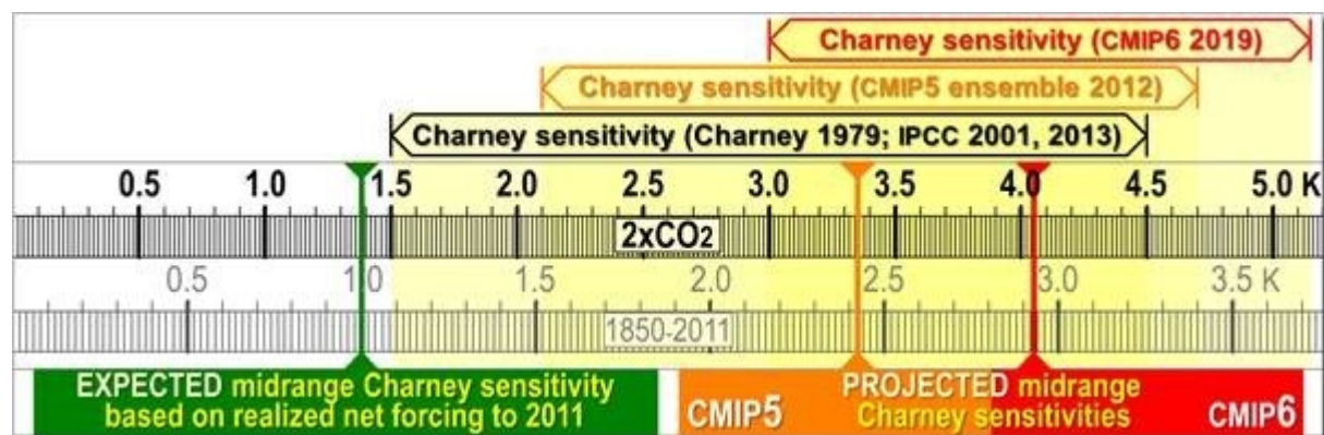
Abbildung 7: Projizierte mittlere Charney-Sensitivitäten (CMIP5 3,35 K orange, CMIP6 4,05 K rot). Sie liegen um das 2,5 bis 3-fache über den 1,4 K (grün), die erwartet werden können bei der gegebenen beobachteten globalen Erwärmung von 0,75 K von 1850 bis 2011 und einem erkannten anthropogenen Antrieb von 1,87 W/m 2 bis 2011. Der gesamt-anthropogene Antrieb von 2,5 W/m 2 bis 2011 wird auf die 3,45 W/m 2 geschätzten Antriebe skaliert als Reaktion auf eine CO 2 -Verdoppelung. Folglich würde die Charney-Sensitivität nach CMIP6 von 1850 bis 2011 eine Erwärmung um fast 3 K implizieren, also drei mal so hoch wie die zu erwartende und vier mal so hoch wie die beobachtete Erwärmung von 0,75 K.
