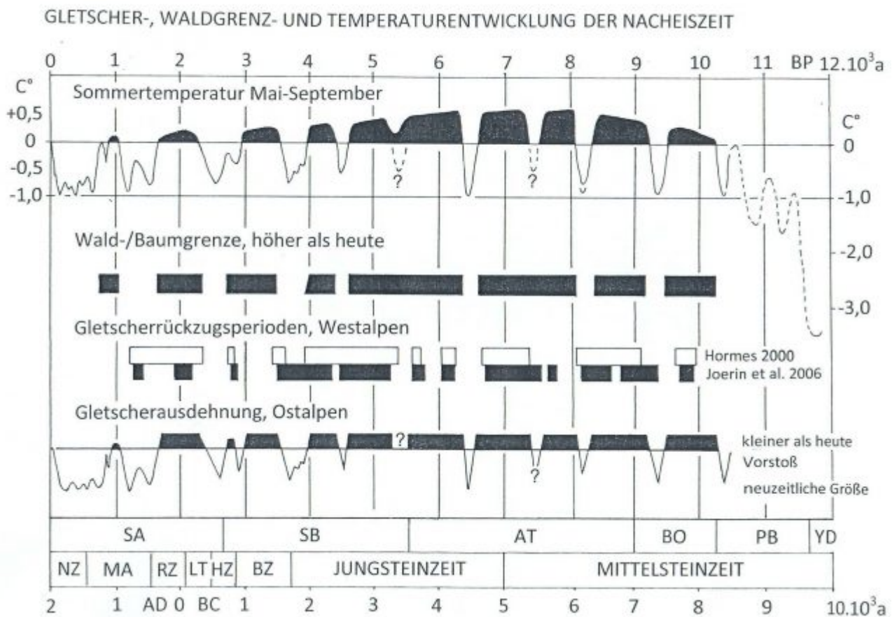
Bild 1: Sommertemperatur, Wald-/Baumgrenze, Gletscherrückzugsperioden Westalpen, Gletscherausdehnung Ostalpen, Grafik aus S. 238 des besprochenen Buchs von G. Patzelt.
