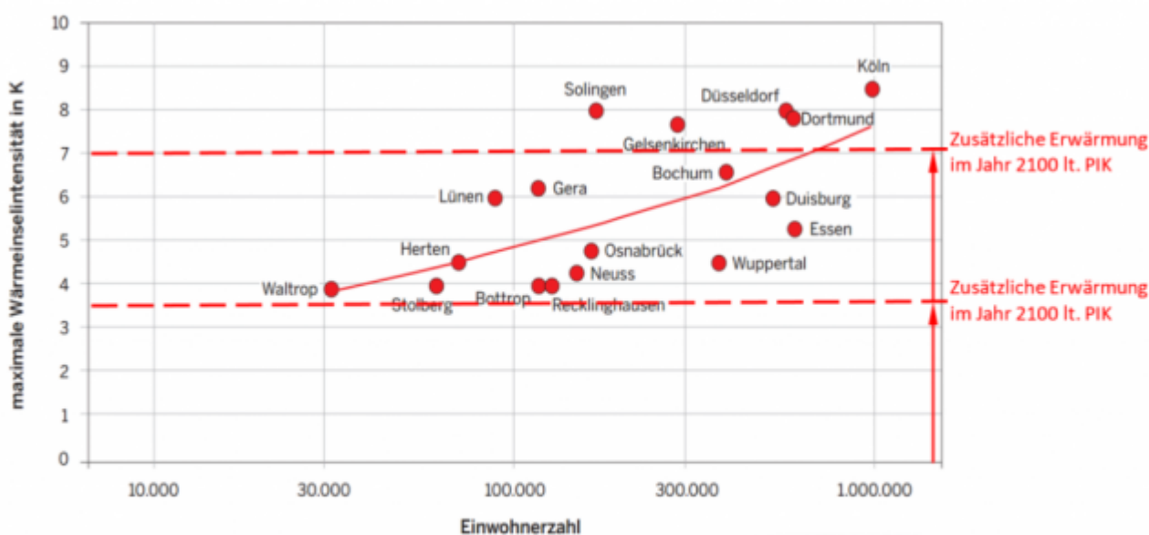
Abbildung 32: Maximale Wärmeintensitäten in Abhängigkeit von der Einwohnerzahl für ausgewählte Städte überwiegend aus NRW (KUTTLER 2011)
