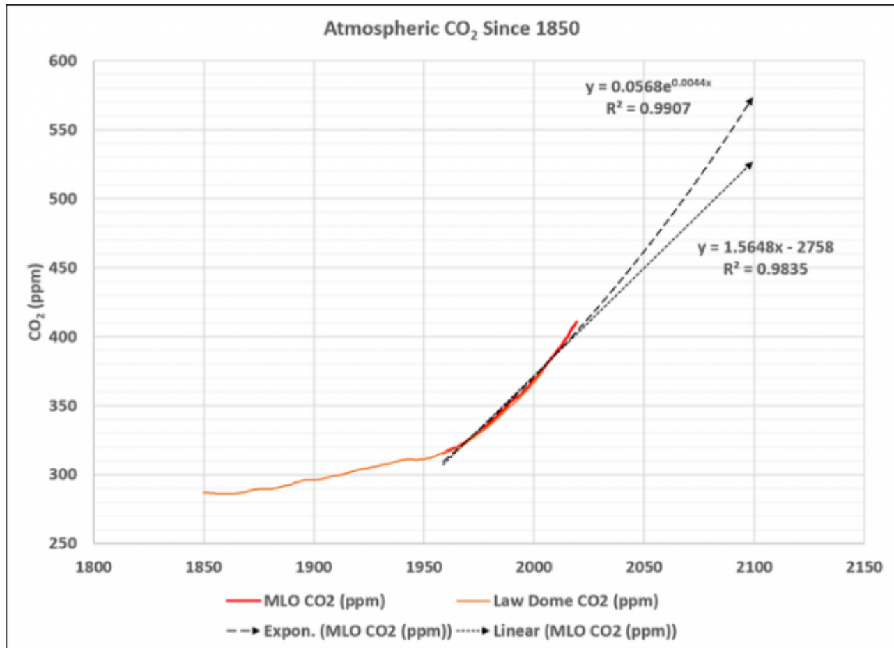
Abbildung 6: Atmosphärisches CO 2 , gemessen am Mauna Loa Observatorium (MLO, NOAA/ESRL) und der Eisbohrkern DE08 vom Law Dome, Antarktis (MacFarling-Meure, 2006).
