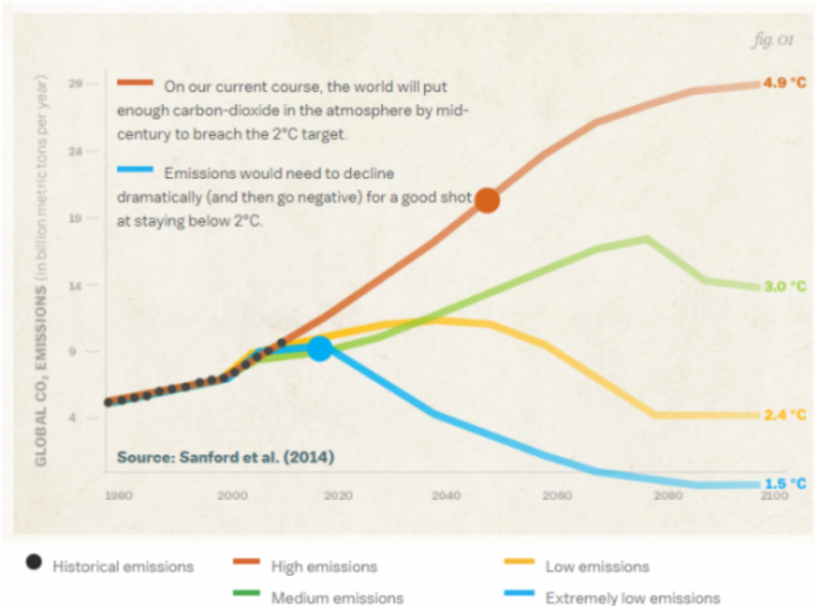
Abbildung 3: Die 2,0°C-Grenze (Vox)
