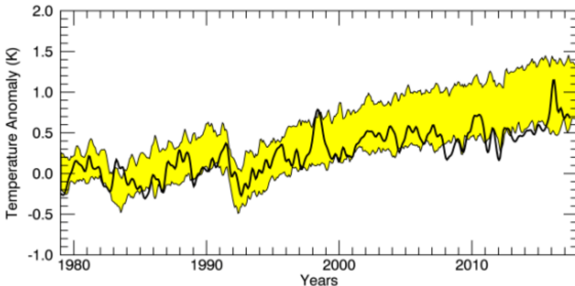
Abbildung 13: Die Modelle haben sich nicht verbessert. Vergleich des RSS V4.0 MSU/AMSU-Datensatzes der Temperatur mit den CMIP5-Klimamodellen. Das gelbe Band ist das Wahrscheinlichkeits-Band 5% bis 95%. Abgesehen vom jüngsten El Nino, war RSS ( Remote Sensing Systems ) kühler als über 95% aller Modelle. Der prädiktive Zustand ist nach 2005 ...
