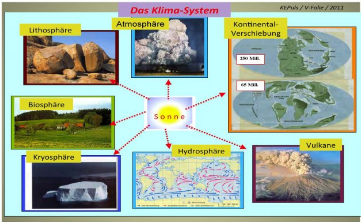
Abbildung 4 Das Klima-System
