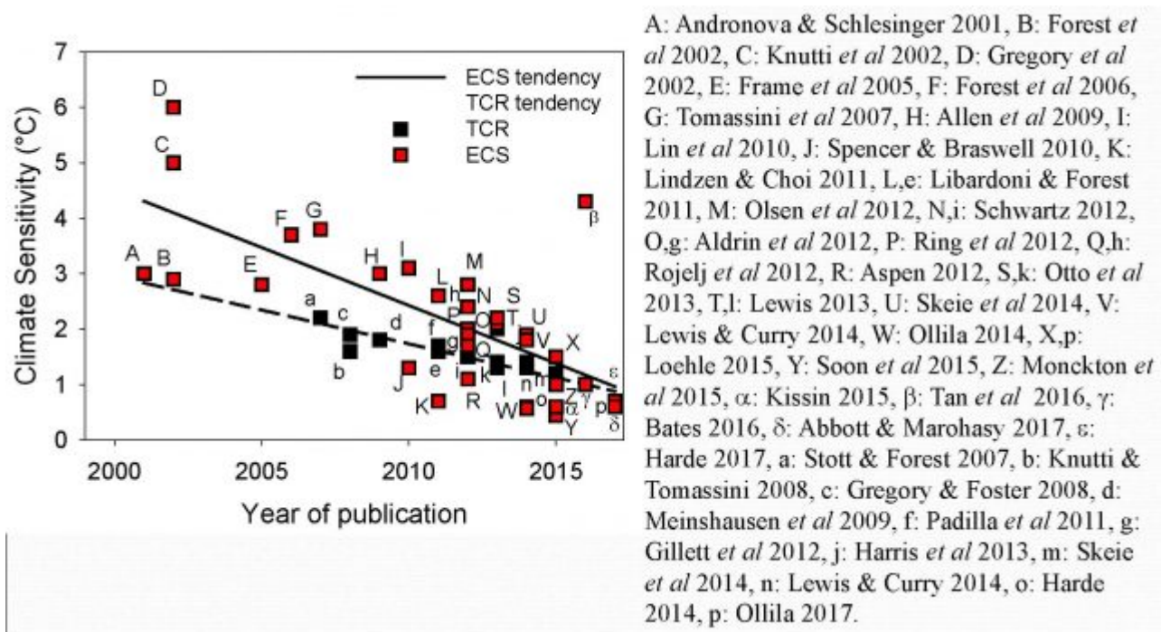
Bild 1: Klimasensitivitätswerte von ECS und TCR in Abhängigkeit vom Veröffentlichungsdatum. Der TCR-Trend hin zu tieferen Werten als 1 °C ist unverkennbar [8], [9]. Damit wäre übrigens das 1,5 °C – Ziel des Pariser Klima-Abkommens längst erreicht und das Abkommen überflüssig geworden.
