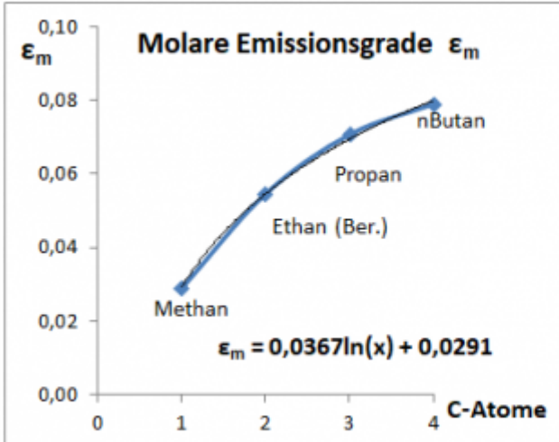
Abb. 5: Emissionsgrade \epsilon_{Gas}(n) für Methan (CH4), Propan (C3H8) und nButan (C4H10) in Abhängigkeit von der Molmenge
