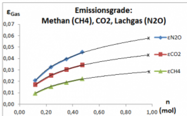
Abb. 1: Gefundene und berechnete Emissionsgrade von Methan, \text{CO}_2 und Lachgas für 0,1 - 1,0 mol
