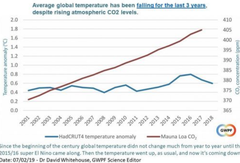
Abbildung 2: Obwohl die CO 2 -Konzentrationen der Luft seit 2001 kontinuierlich angestiegen sind, hat sich die globale Durchschnittstemperatur nur wenig verändert
