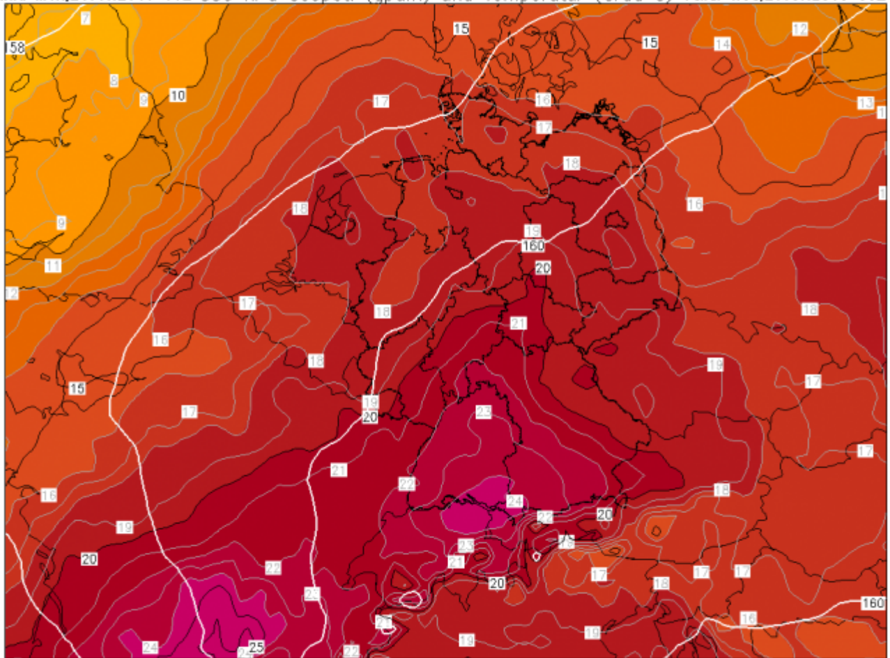
Abb. 1: Simulierte Temperatur- und Druckverteilung im 850-hPa-Niveau über Mitteleuropa für Mittwoch, den 26. Juni
