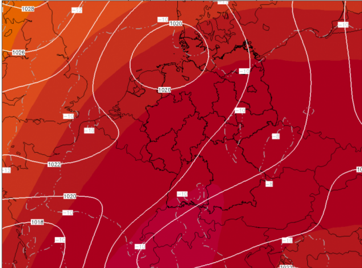
Abb. 2: Simuliertes Geopotential im 500-hPa-Niveau (farbige Konturen) und Bodenluftdruck (dünne weiße Linien) über Mitteleuropa für den 26. Juni
