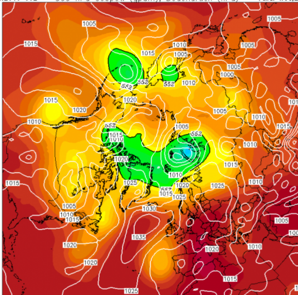
Abb. 4: Wie Abb. 2, aber über der gesamten Nordhemisphäre
