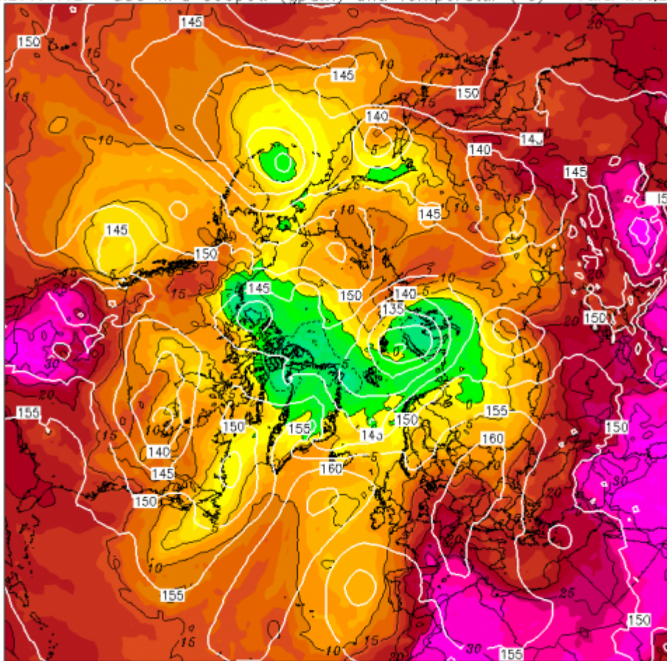
Abb. 3: Wie Abb. 1, aber über der gesamten Nordhemisphäre
