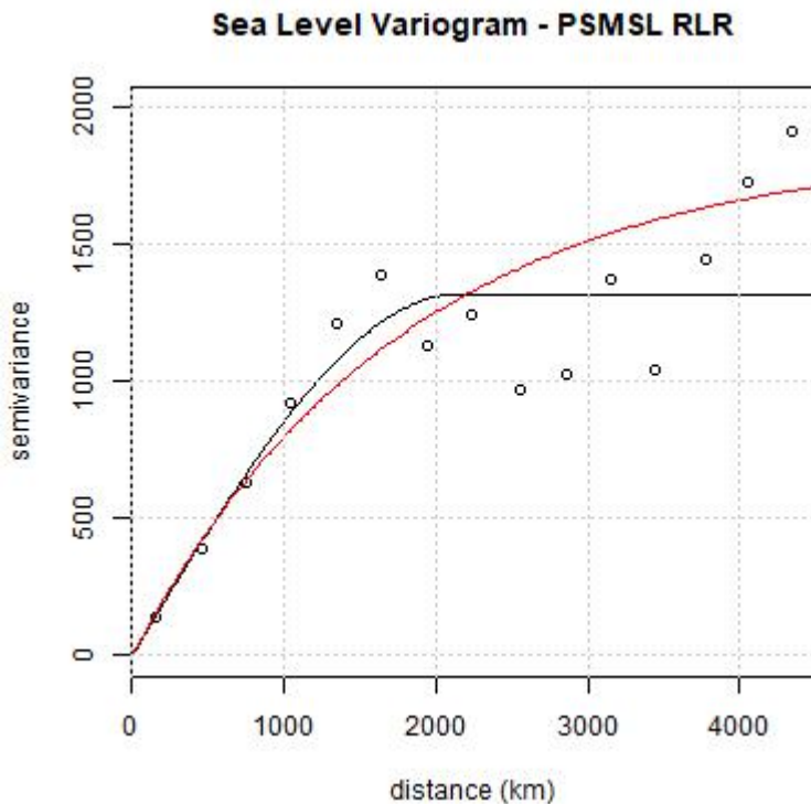
Abbildung 3: SLR-Variogramm. Schwarz: sphärischer Fit , rot: exponentieller Fit
