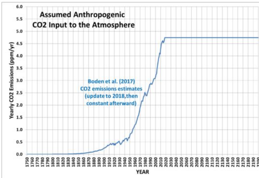
Abbildung 1: Vermuteter jährlicher CO 2 -Eintrag in die Modell-Atmosphäre
