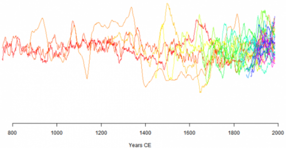
Bild 1 Pages2k-Projekt: Verlauf aller Temperaturproxis Nordamerika seit 1200. Quelle: Pages2k Viewer (Screenshot vom Autor)
