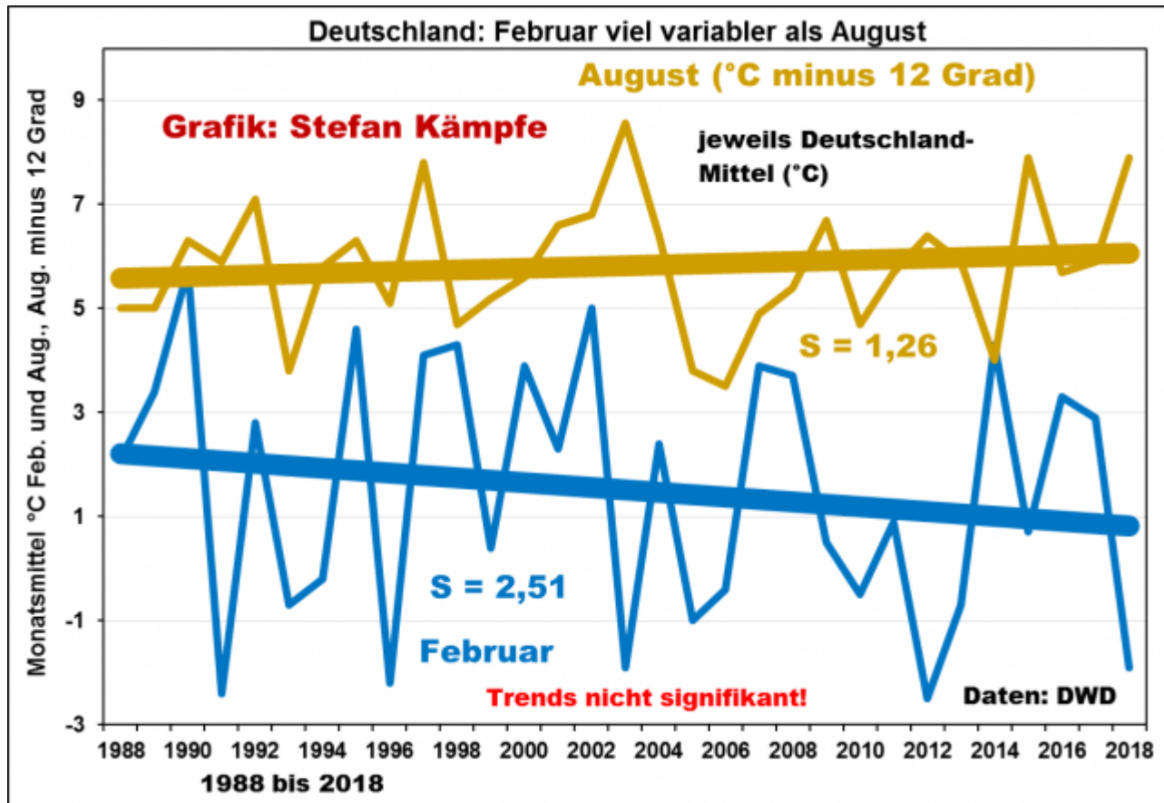
Abbildung 4: Februar-Monatsmittelterperaturen streuen enorm. Zum Vergleich ist das August-Mittel, zur besseren Veranschaulichung um 12 Grad abgesenkt, mit dargestellt; Trend und Streuung verändern sich dadurch nicht.
