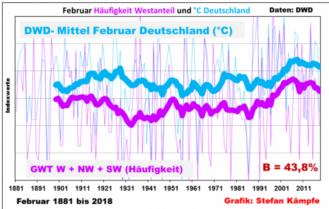
Abbildung 2: Am Ende 20. Jahrhunderts stiegen die Februar-Temperaturen stark an, weil Westwetterlagen deutlich häufiger wurden. In den sehr milden Februar-Monaten 1990 und 1997 traten sie an allen 28 Februartagen auf! Die sehr unterschiedlichen Größen Lufttemperatur und Westlagenhäufigkeit mussten zur besseren Veranschaulichung in Indexwerte umgerechnet werden.
