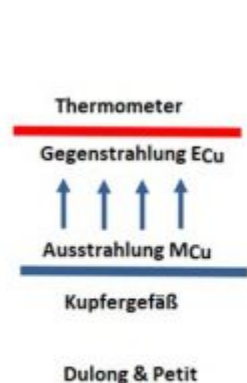
Abb. 5: Ohne Seitenwand Gegenstrahlung: E_{Cu} = M_{Cu}
