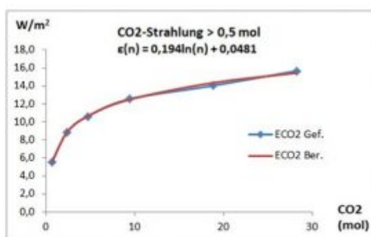
Abb. 16: Berechnete und gefundene CO 2 -Strahlungswerte nach Gl. 9/8.2
