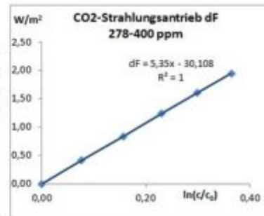
Abb. 18: Zunahme des CO 2 -Strahlungsantriebs von 1,95 W/m 2 seit 1750 nach IPCC-Gl. 10
