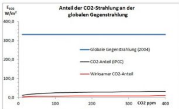
Abb. 1: Die erdnahe CO 2 -Strahlung
