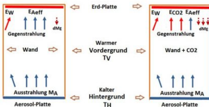
Abb. 6: Mit Seitenwand W Gegenstrahlung: E_W + E_{Aeff} > M_A
