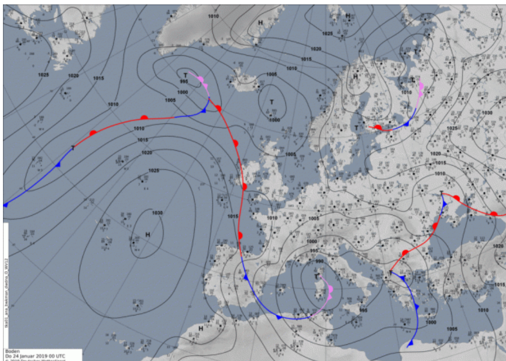
Abb.1 DWD-Bodenwetterkarte 24.01.2019 [2]
