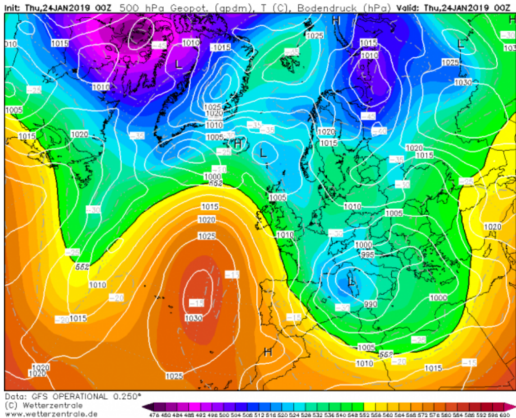
Abb.2 Höhenwetterkarte 500 hPa 24.01.2019 [2]
