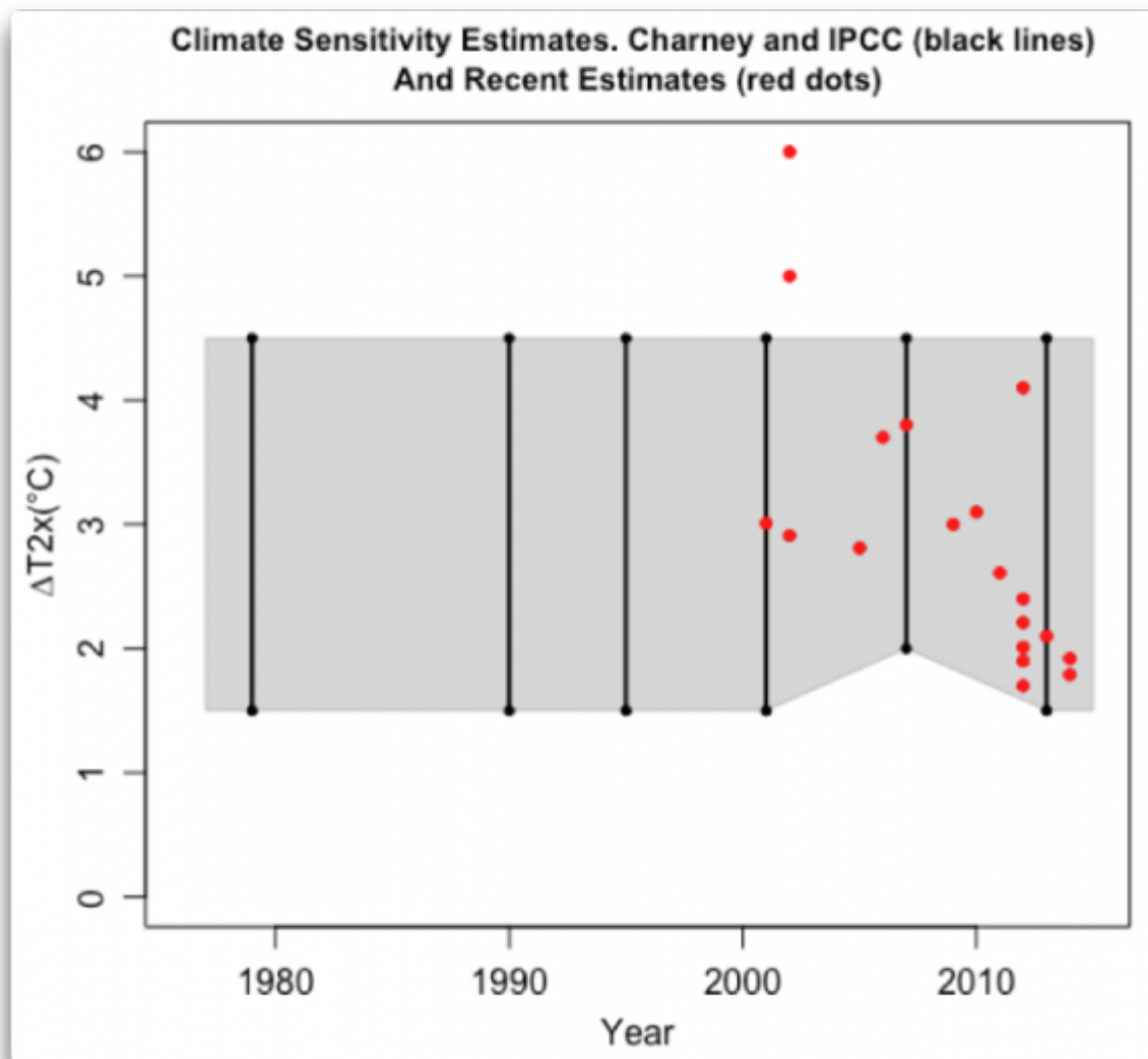
Abbildung 5: Änderungen über die Zeit der Schätzung des Klimasensitivitäts-Parameters „lambda“. „ \Delta T_{2x}(\text{°C}) “ ist die erwartete Temperaturänderung in Grad Celsius bei einer Verdoppelung des atmosphärischen \text{CO}_2 -Gehaltes, von welcher man annimmt, dass sie das Forcing um 3,7 \text{ W/m}^2 verstärken wird. Mit den Abkürzungen FAR, SAR, TAR, AR4, AR5 sind die fünf Zustandsberichte des IPCC gemeint, welche eine Zustandsbeschreibung des Status' der Klimawissenschaft zum jeweiligen Zeitpunkt der Berichte sind. Rote Punkte zeigen die aktuellsten individuellen Schätzungen der Klimasensitivität.
