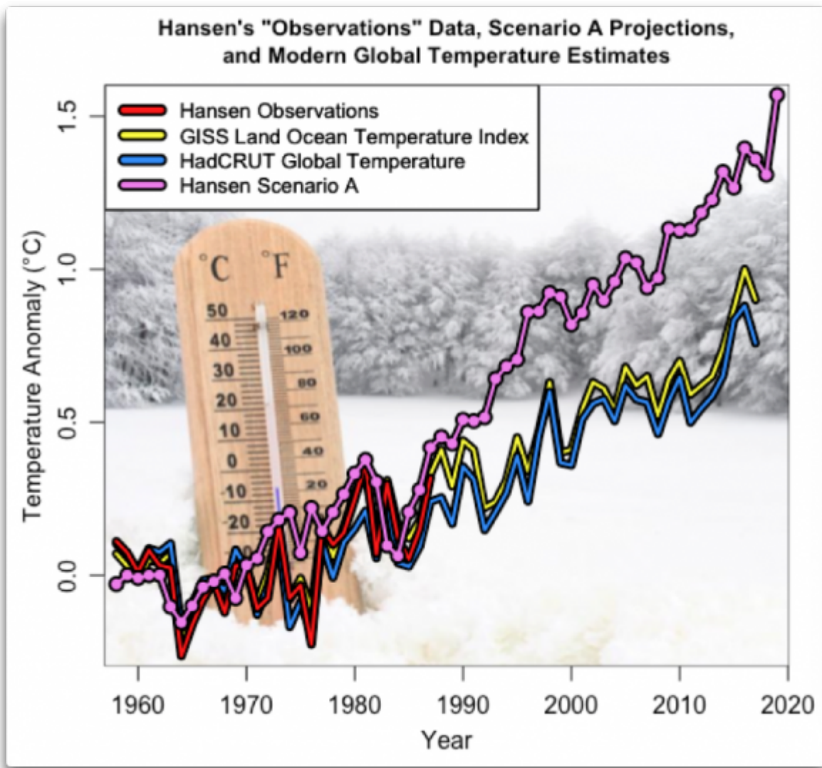
Abbildung 4: Die in Hansens Graphik oben als „Beobachtungen“ bezeichnete Linie zusammen mit seiner Szenario A-Schätzung im Vergleich zu aktuellen Temperatur-Schätzungen. Alle gemessenen Daten sind als Anomalie vom Mittel der Jahre 1951 bis 1980 dargestellt.
