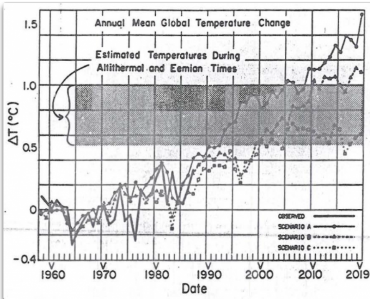
Abbildung 1: Original-Bildunterschrift: Abbildung 3. Jährliche mittlere globale Lufttemperatur, berechnet für die Spurengas-Szenarien A, B und C. (Szenario A nimmt weiter wie seit 20 Jahren steigende Emissionen, Szenario B friert die Emissionen auf dem jetzigen Stand ein, Szenario C zeigt drastisch reduzierte Emissionen von 1990 bis 2000). Der schattierte Bereich repräsentiert eine Schätzung der globalen Temperatur während des Höhepunktes der gegenwärtigen und von früheren Interglazial-Perioden, jeweils etwa vor 6000 und 120.000 Jahren vor heute. Der Nullpunkt der Messungen ist das Mittel des Zeitraumes 1951 bis 1980, der Nullpunkt für das Modell ist das Mittel des Kontroll-Laufes.
