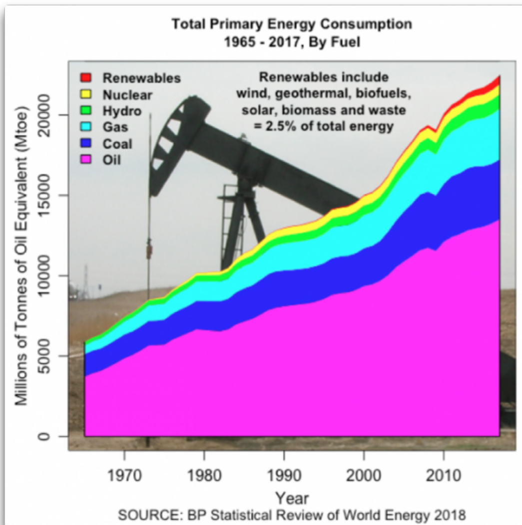
Abbildung 1: Globaler Gesamt-Primär-Energieverbrauch 1965 bis 2017
