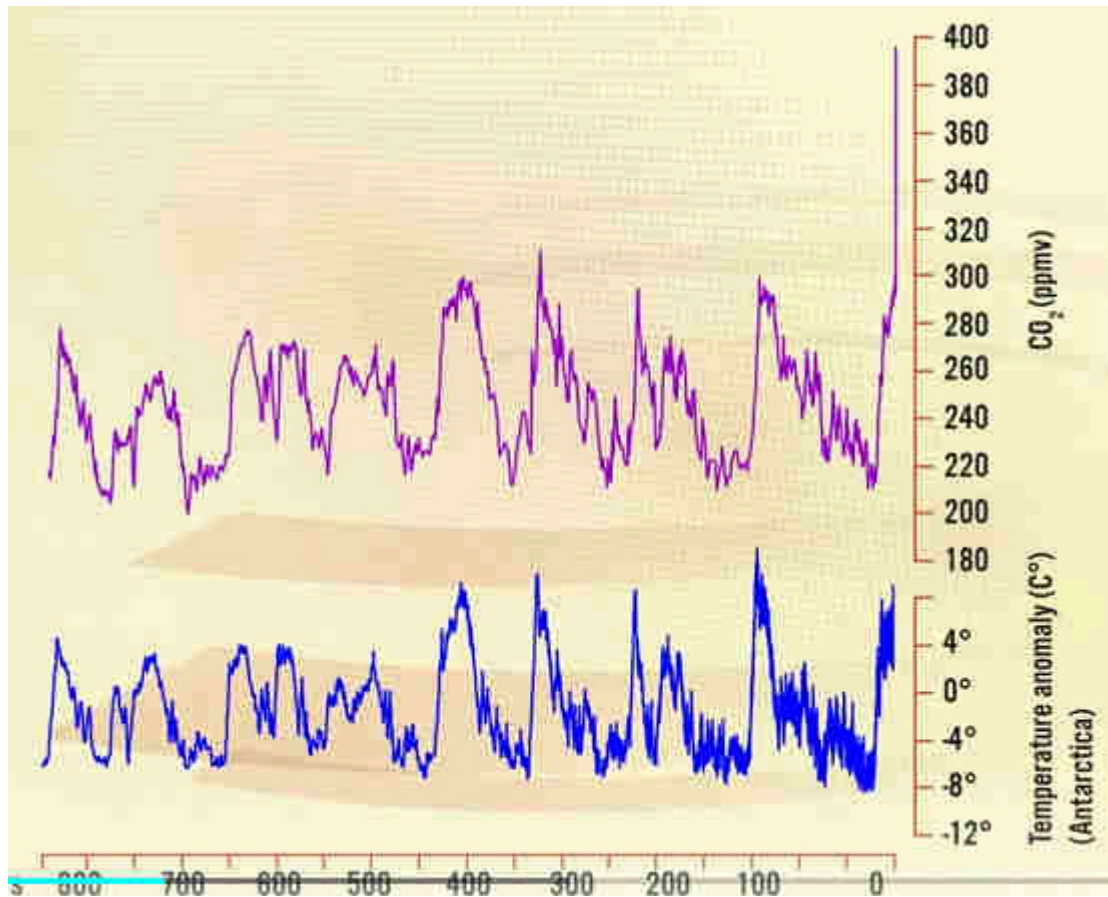
Abb.2: Der „fast perfekte“ Gleichlauf von Temperatur und CO 2 in Eisbohrkernen liessen Al Gore mit seinem Film « Eine unbequeme Wahrheit » an die Ursache CO 2 glauben (Quelle: IPCC).
