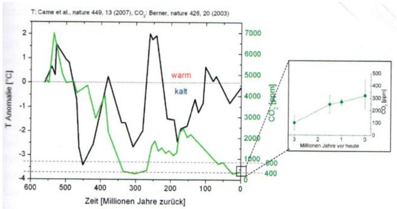
Abb.1: Die Temperatur (schwarz) änderte sich völlig unabhängig vom CO 2 -Gehalt (grün) in der Atmosphäre !
