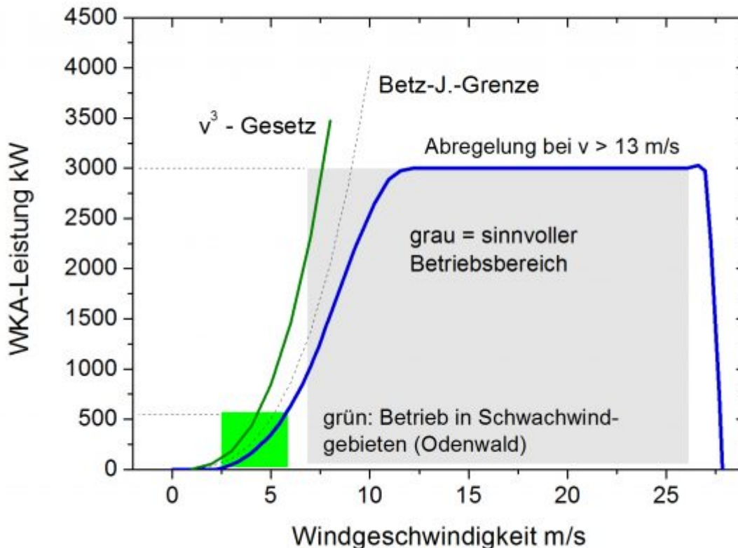
Windradkennlinie: entspricht der Enercon E 115
