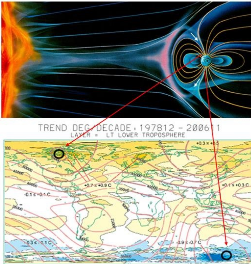
Abb.18, Quelle, zeigt vereinfacht die Wechselwirkung des IPF mit dem Erdmagnetfeld (weiße Pfeile) und den Verlauf der Feldlinien im solaren Minimum (wie derzeit). Darunter sind die globalen Temperaturanomalien in der Fläche für den Zeitraum 12/1978 – 11/2006 zu sehen. Am magnetischen Nordpol (Kreis), wo die Feldlinien und somit die geladenen Partikel einfließen, kommt es zu einer Temperaturerhöhung und am Südpol, wo die Feldlinien heraustreten, also keine Partikel einfließen, kommt es zu einer Temperaturabnahme.
