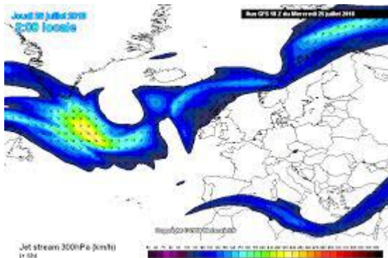
Abb.7,Quelle, zeigt oben blau eingefärbt (je nach Windgeschwindigkeit) den PFJ. Darunter den Teil eines anderen globalen Windsystems, des Subtropenjetstreams, Ende Juli 2018 (26.07.).
