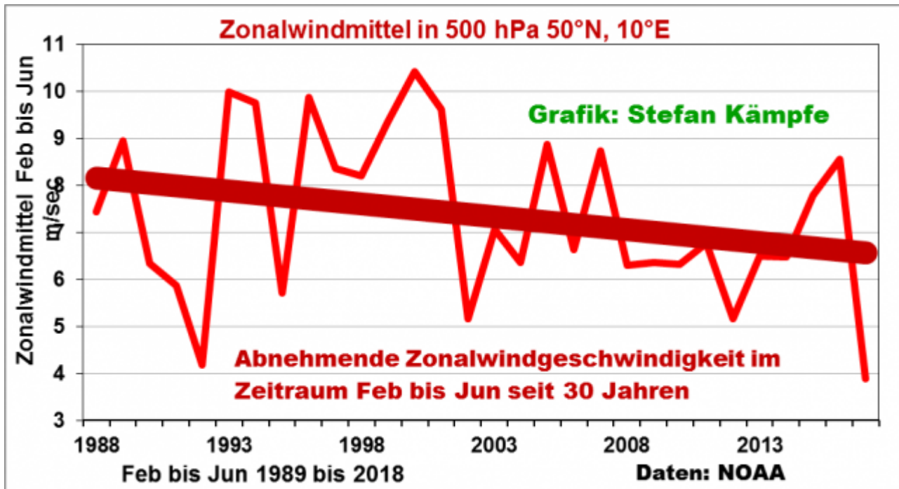
Abbildung 11: Seit 30 Jahren wird der Zonalwind schwächer und erreichte in diesem Betrachtungszeitraum seinen niedrigsten Wert im Extremwetterjahr 2018.
