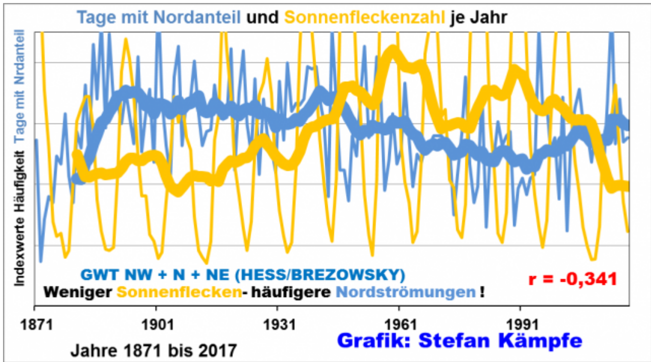
Abbildung 9: Langfristig treten in Mitteleuropa mehr nördliche Großwetterlagen auf, wenn die Sonnenfleckenanzahl geringer ist – so auch gegenwärtig. Aber nur im Frühling und Herbst sind fast alle diese Lagen
