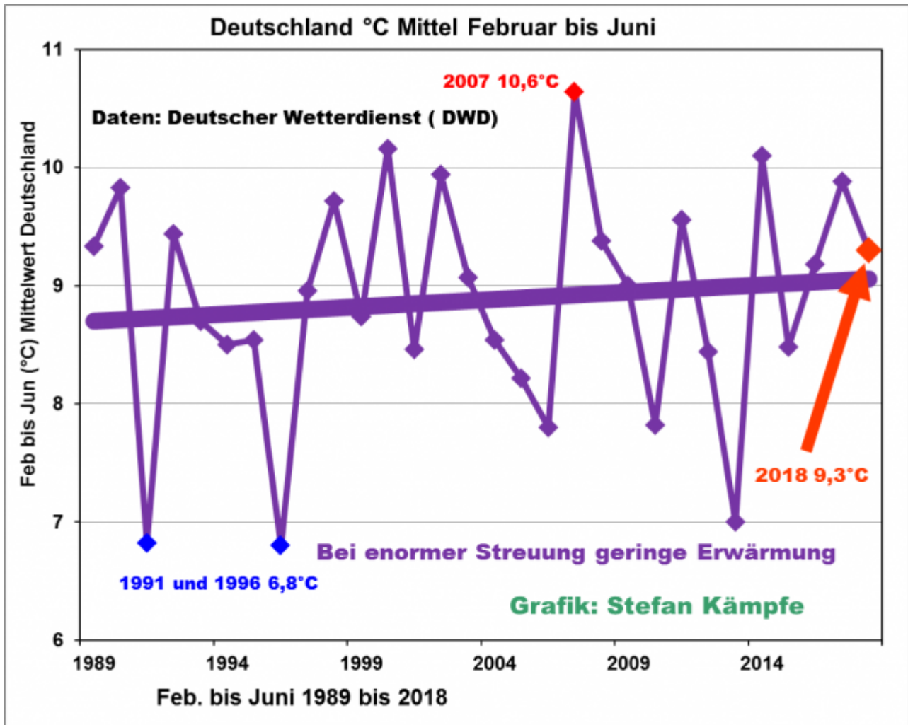
Abbildung 4: Nur leichte Deutschland-Erwärmung im Zeitraum von Februar bis Juni seit 1989. Im Jahr 2018 lag dieser Zeitraum mit nur 9,3°C lediglich im oberen Mittelfeld; weit entfernt von den wärmsten Werten.
