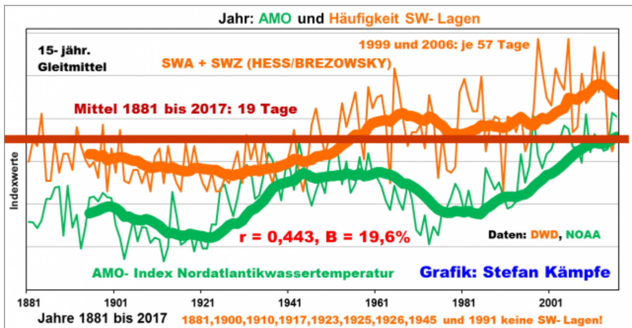
Abbildung 1: Seit 1881, dem Beginn der Erstellung halbwegs verlässlicher Wetterkarten, hat sich die Häufigkeit der in Deutschland stark erwärmend wirkenden Südwestlagen merklich erhöht. Außerdem erwärmte sich der Nordatlantik, wobei es eine schwächere Warmphase um 1900, eine stärkere um 1945 und eine aktuelle gibt. Die Kurvenverläufe der gleitenden Mittelwerte (fette Kurven) ähneln sich; wobei die AMO fast 20% der Häufigkeitsvariabilität der SW- Lagen erklärt. Fast alle Jahre ganz ohne SW- Lagen traten vor 1950 auf; danach war nur 1991 frei von SW- Lagen.
