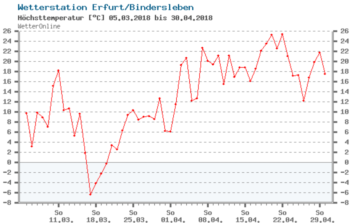
Abb. 2: Rasche Frühlingserwärmung ist in unserem subkontinentalen Klima nicht selten; aber um gut 30 Grad in nur 4 Wochen- das gibt es nur selten und erinnert sehr stark an die klimatischen Verhältnisse in Russland. Quelle: www.wetteronline.de
