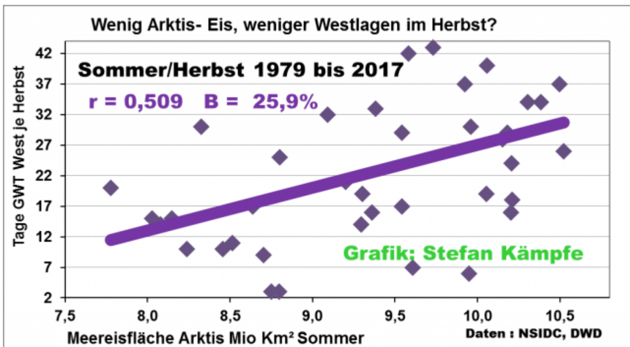
Abbildung 15: War die Arktische Meereis- Ausdehnung im Sommer gering, so wie auch 2018, dann gab es im Herbst tendenziell weniger Westwetterlagen (GWT West, bestehend aus WA, WZ, WS und WW nach der HESS/BREZOWSKY- Klassifikation).
