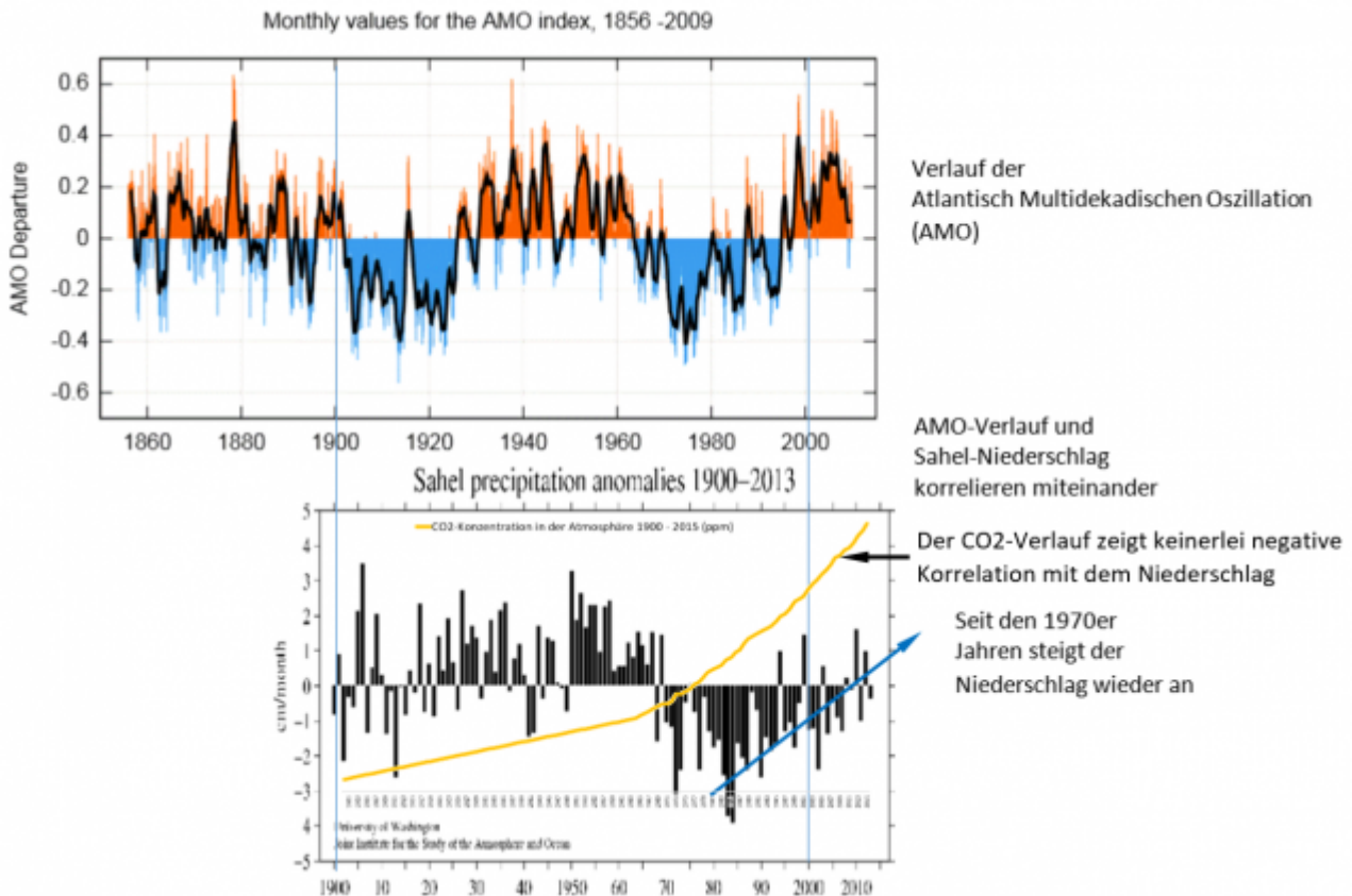
Bild 1 [4] Sahelzone: Zusammenhang zwischen der AMO und dem Niederschlagsverlauf von 1900 – 2010, sowie CO 2 -Konzentrationsverlauf. Vom Autor zusammengesetzt
