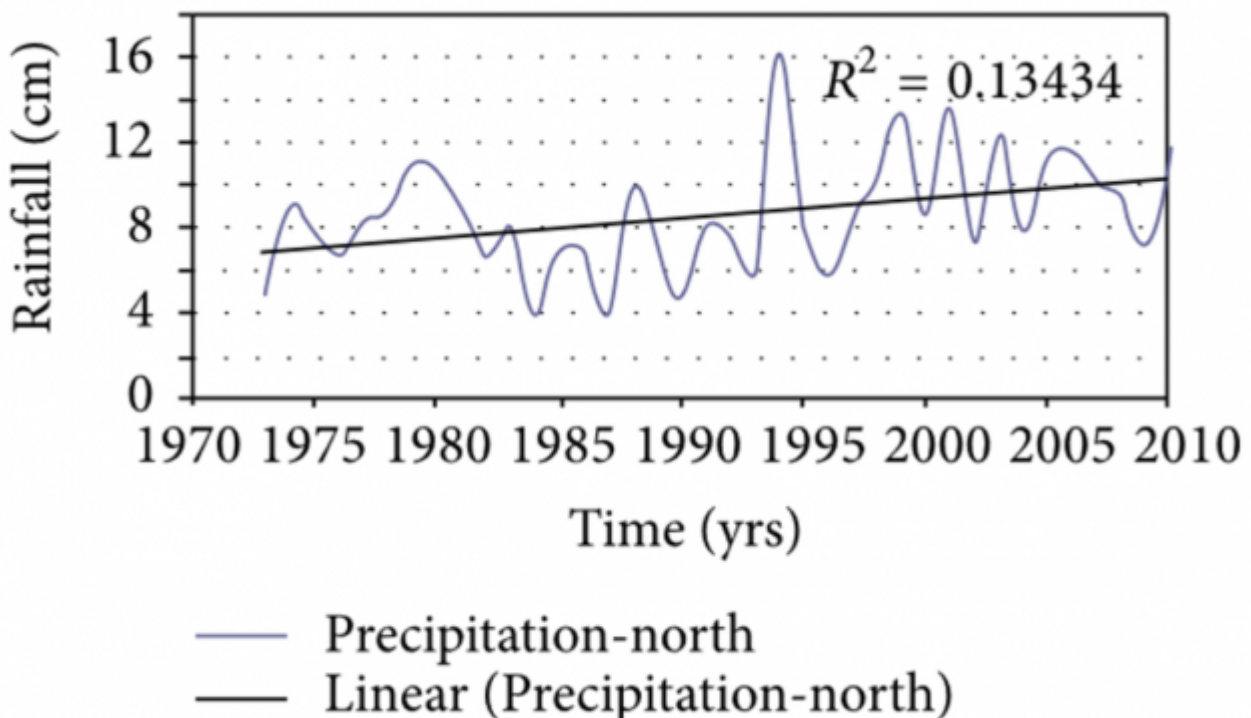
Bild 2 Niederschlagsverlauf im Nordend des Sahel seit 1970 (Teilbild) [12]
