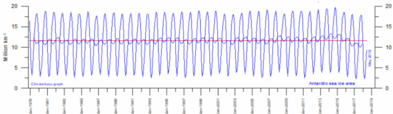
Bild 4 Antarktis, Verlauf der Meereisausdehnung von 1979 bis 5.2018
