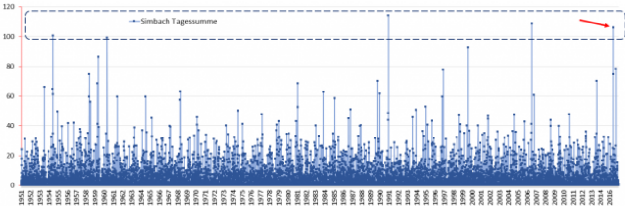
Bild 19 [24] Niederschläge Simbach Tageswerte 1951 – 2016. Vom Autor aus den DWD-Daten mit einer Ergänzung des Niederschlagspegels am 1.6.2016 erstellt (roter Pfeil)
