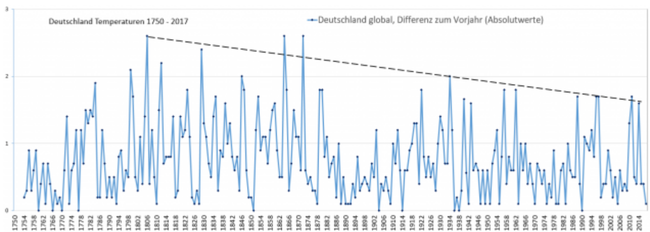
Bild 31 Deutschland Temperatur 1750 – 2018. Absolutwerte der Jahresdifferenz. Grafik vom Autor anhand der DWD-Daten erstellt
