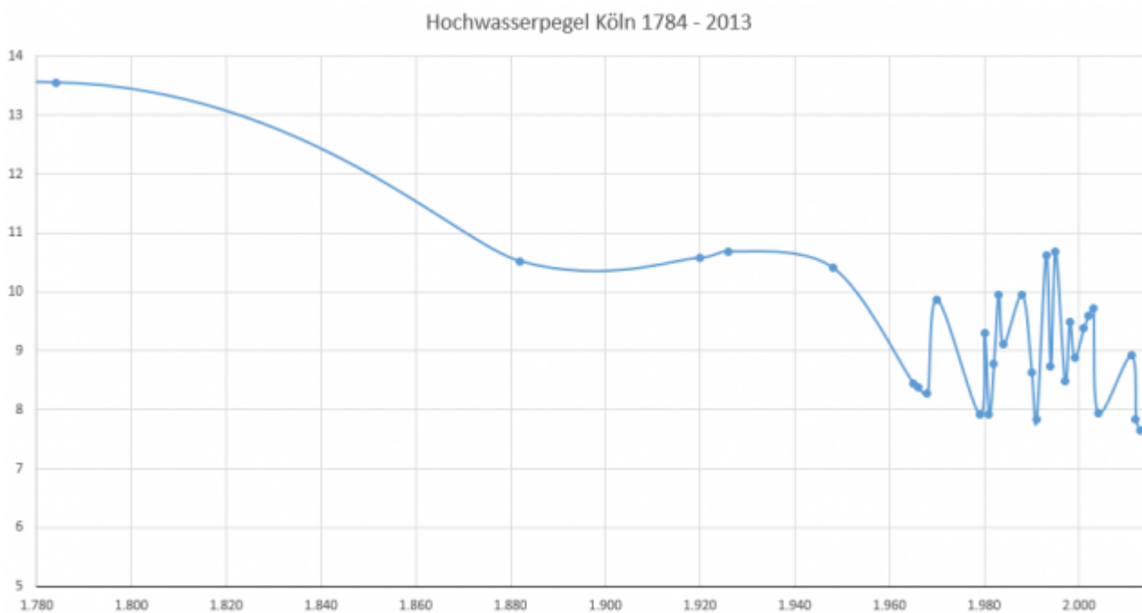
Bild 21 Hochwasserpegel Köln 1784 – 2013 lt. Daten der Stadtentwässerungsbetriebe Köln AöR (Grafik aus den Tabellendaten vom Autor erstellt). Y-Achse: Rheinpegel (m)
