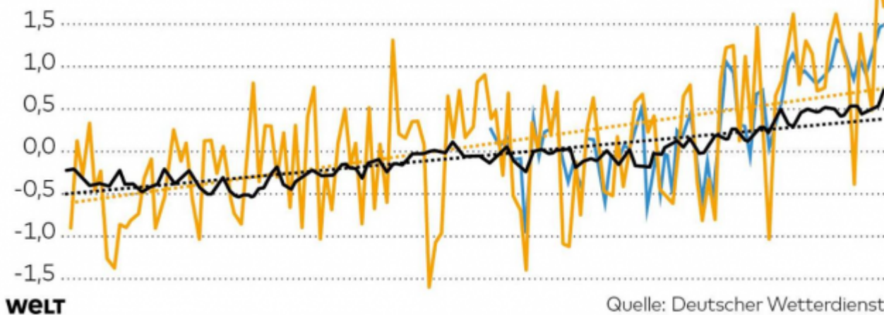
Bild 6 Temperatur-Verlaufvergleich Deutschland und Welt global [2]
