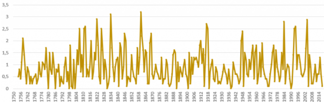
Bild 33 Deutschland Temperatur Sommer 1750 – 2018. Absolutwerte der Jahresdifferenz. Grafik vom Autor anhand der DWD-Daten erstellt
