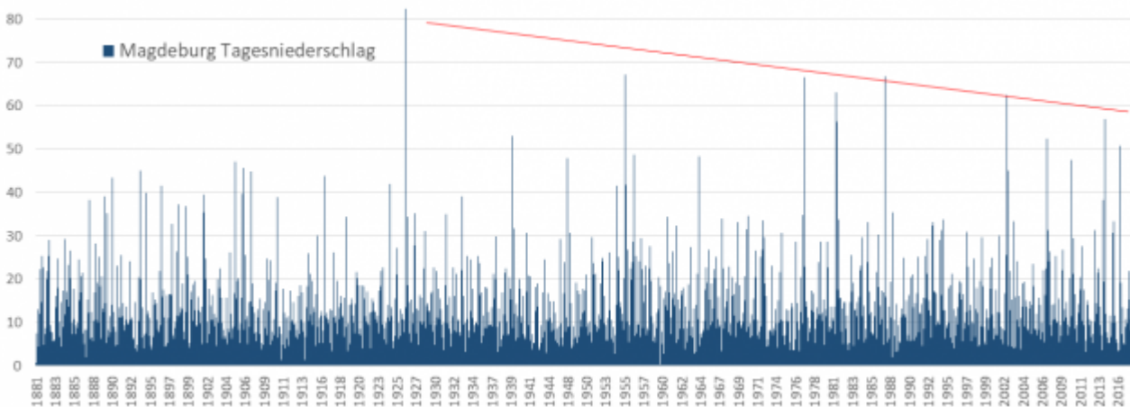
Bild 17 [18] Magdeburg, Tagesniederschlag 1881 – 25.05.2018. Quelle: DWD Daten Station 3126. Grafik vom Autor erstellt
