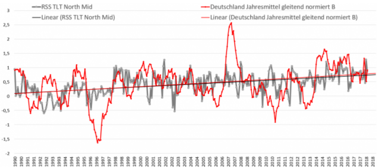
Bild 8 RSS-Satellitendaten North Mid und Deutschland DWD-Stationsdaten seit 1990. Grafik vom Autor erstellt
