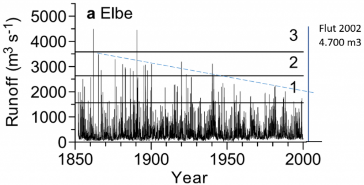
Bild 20 Elbe, Fließmengen 1850 – 2002. Wert der Flut 2002 von 4.700 \text{m}^3 vom Autor nach den Angaben in der Studie ergänzt. Quelle: MUDELSEE ET AL.: EXTREME FLOODS IN CENTRAL EUROPE
