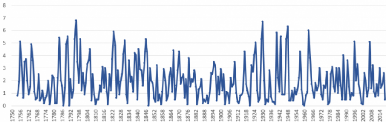
Bild 32 Deutschland Temperatur Winter 1750 – 2018. Absolutwerte der Jahresdifferenz. Grafik vom Autor anhand der DWD-Daten erstellt
