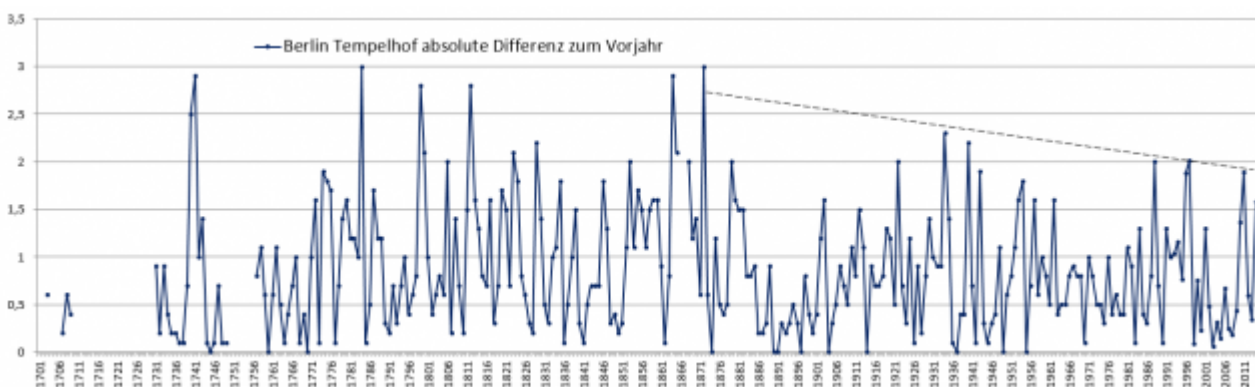
Bild 34 Langzeitreihe Berlin-Tempelhof. 1701 – 2012. Absolutwerte der Jahresdifferenz. Grafik vom Autor anhand der DWD-Daten erstellt
