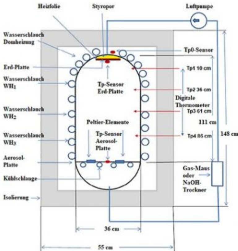
Abbildung 2: Links: Schematischer Aufbau des Experimentes; Rechts: von oben nach unten: Erd-Platte, Aluminiumröhre und Aerosol-Platte
