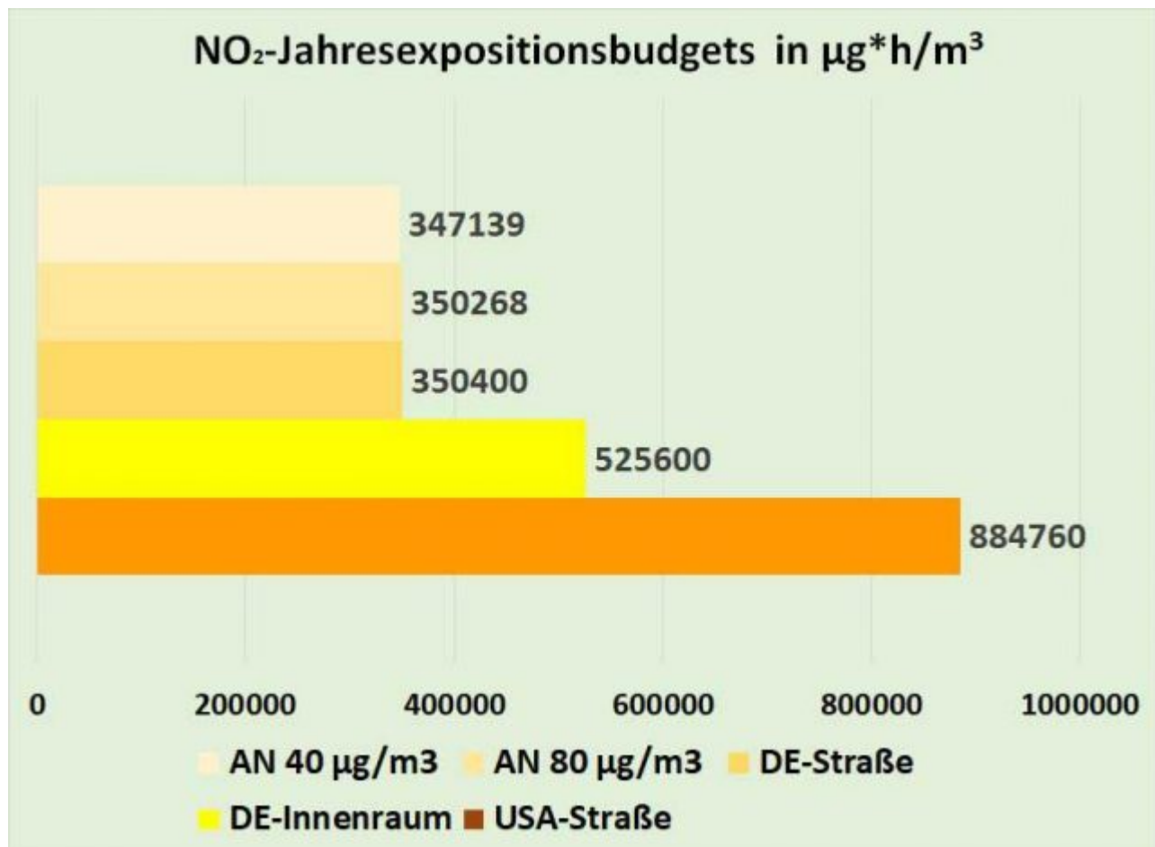
Bild 7. Berechnung der Jahresexpositionsbudgets für zwei Arbeitnehmer in Straßen mit 80 bzw. 40 \mu\text{g}/\text{m}^3 \text{NO}_2 bei einem \text{NO}_2 -Innenraumwert von 40 \mu\text{g}/\text{m}^3
