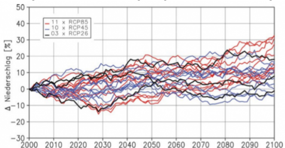
Bild 10 [7] Simulationsergebnisse Niederschlagsmenge Winter für Hamburg Kleine Erkenntnisgewinne sind jedoch erkennbar. Diese Ansammlung von Klimaintelligenz kam dahinter, dass die EEG-Stromversorgung wohl vom Wetter abhängt:
