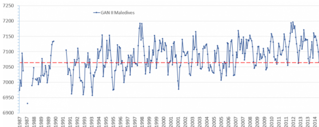
Bild 3 Verlauf des Seepiegels bei den Malediven 1983 – 2014. Bild vom Autor aus den Daten erstellt und ergänzt. Datenquelle: PSMSL Data Explorer
