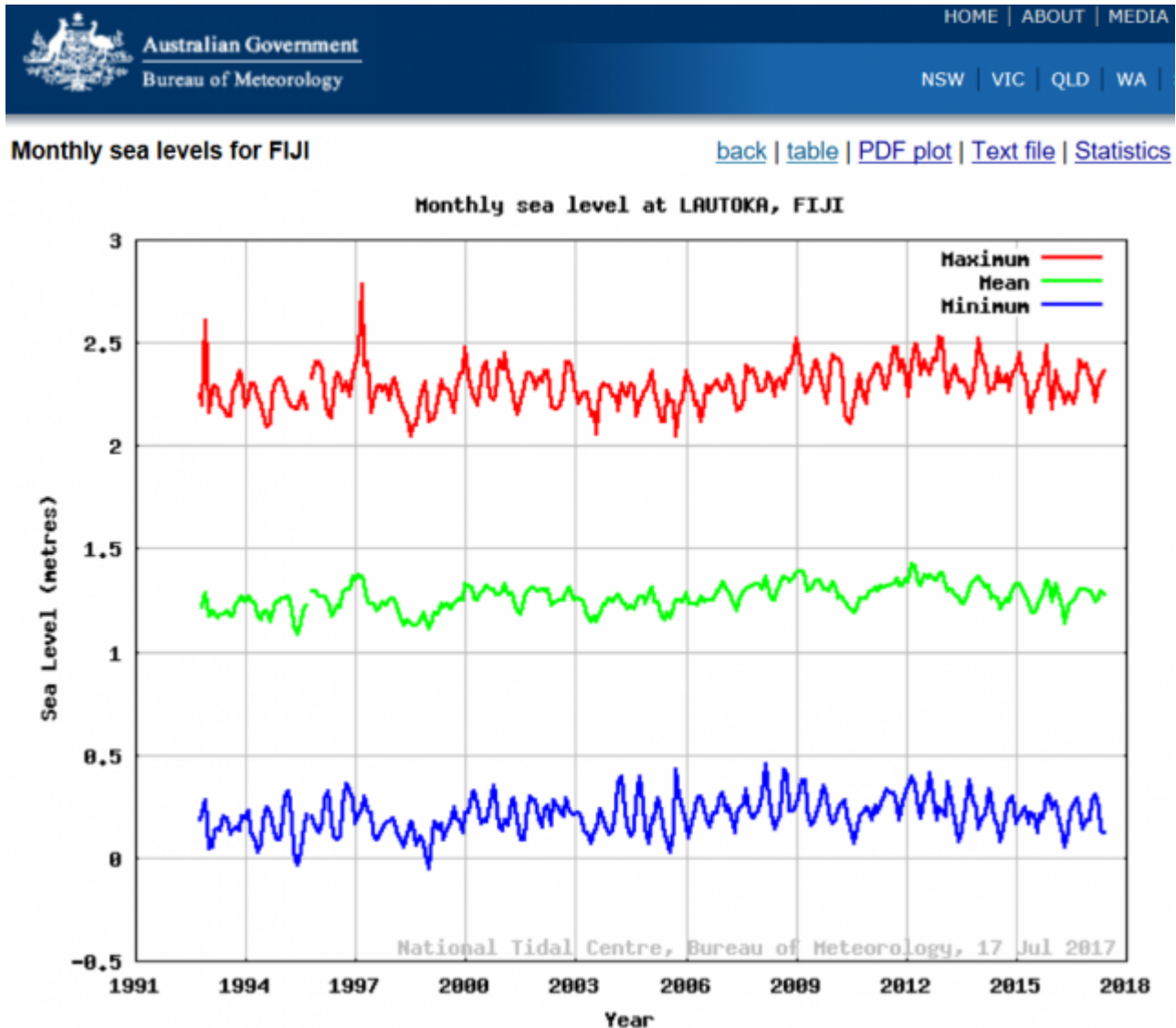
Bild 11 Pegelverlauf Fidji von Ca. 1993 – Juli 2017
