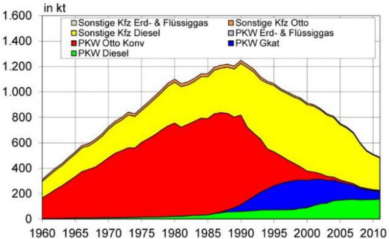
Bild 4. Die Aufschlüsselung der Anteile der einzelnen Fahrzeugarten an den NO x -Emissionen des Straßenverkehrs bis 2011. Der Anteil der Diesel-PKW lag bei lediglich ca. 30 % (Grafik: [TREM])
