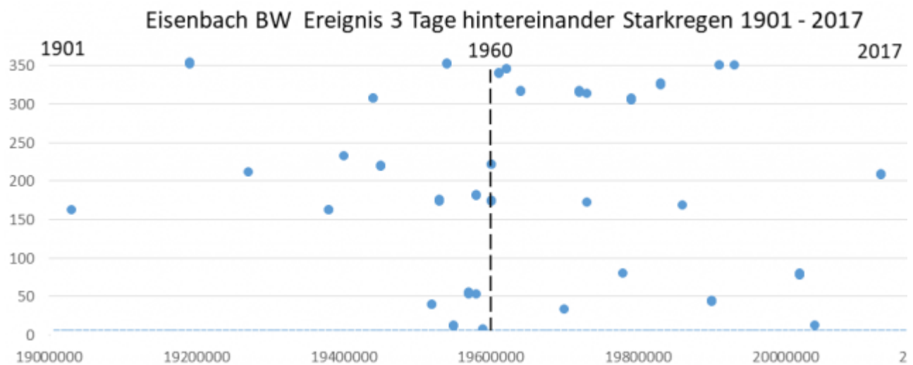
Bild 12 DWD-Messtation Eisenbach, Baden-Württemberg (ID 1176). Ereignistage von 3 Tagen hintereinander auftretendem Starkregen zwischen 1901 – 2017
