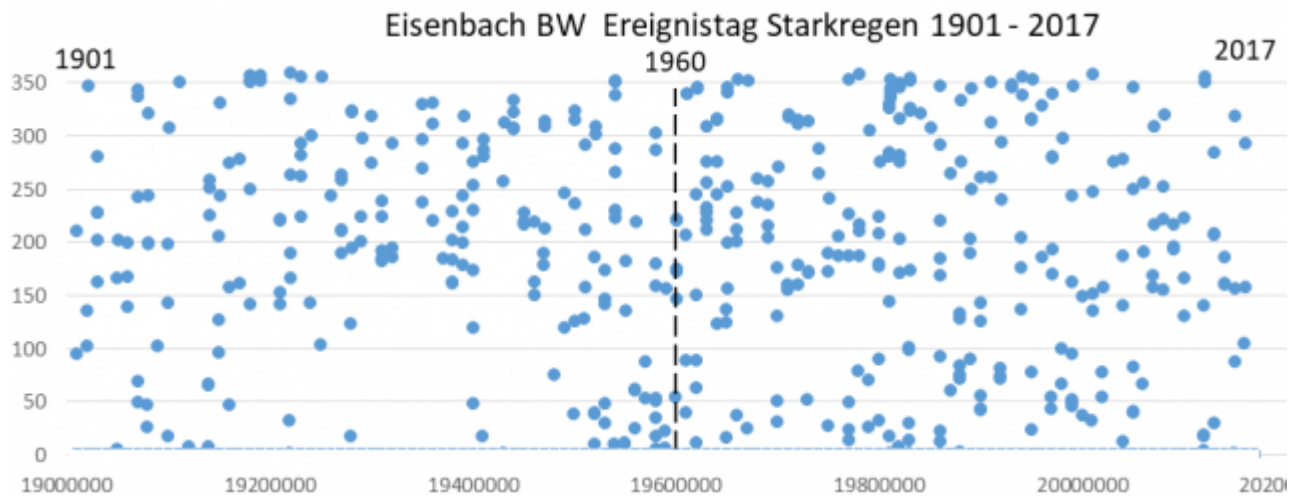
Bild 11 DWD-Messtation Eisenbach, Baden-Württemberg (ID 1176), Tag des Auftretens eines Starkregeneignisses von 1901 – 2017
