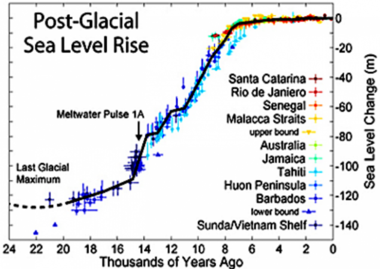
Bild 21 Meeresspegelanstieg seit der letzten Eiszeit
