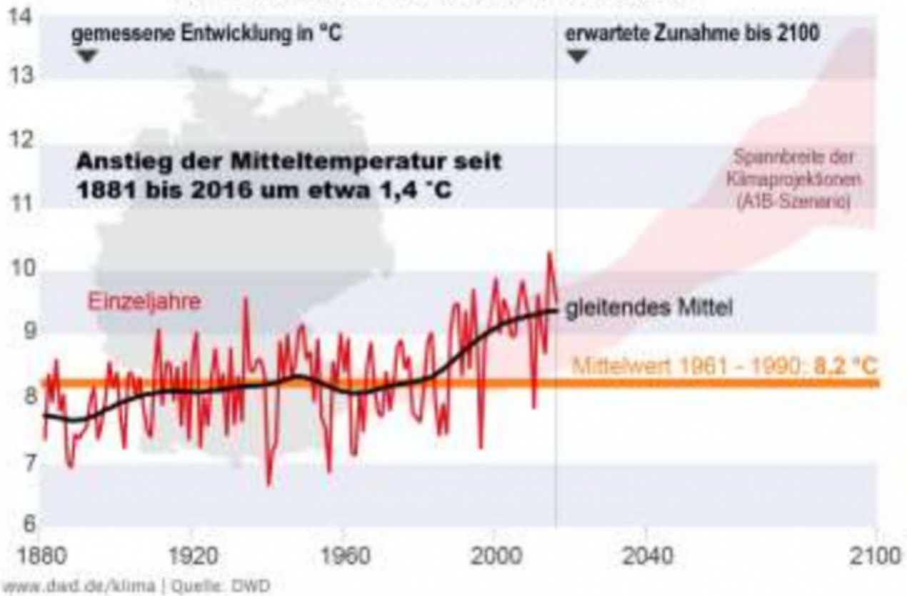
Bild 3-11 [2] Temperatur Deutschland. Grafik im G20-Papier
