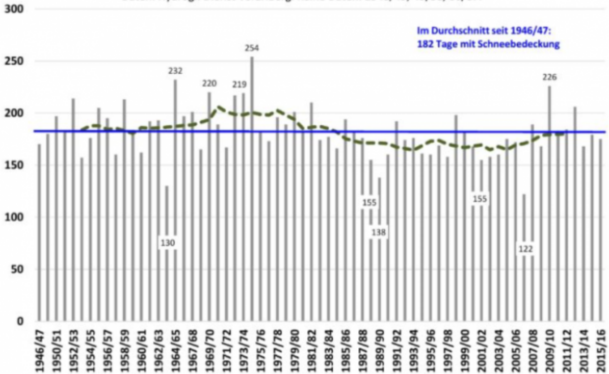
Abb. 2: Der Verlauf der jährlichen Anzahl der Tage mit Schneebedeckung in Damüls von 1946/47 bis 2015/16. Daten: Hydrographischer Dienst Vorarlberg. Grafik: www.zukunft-skisport.at .
