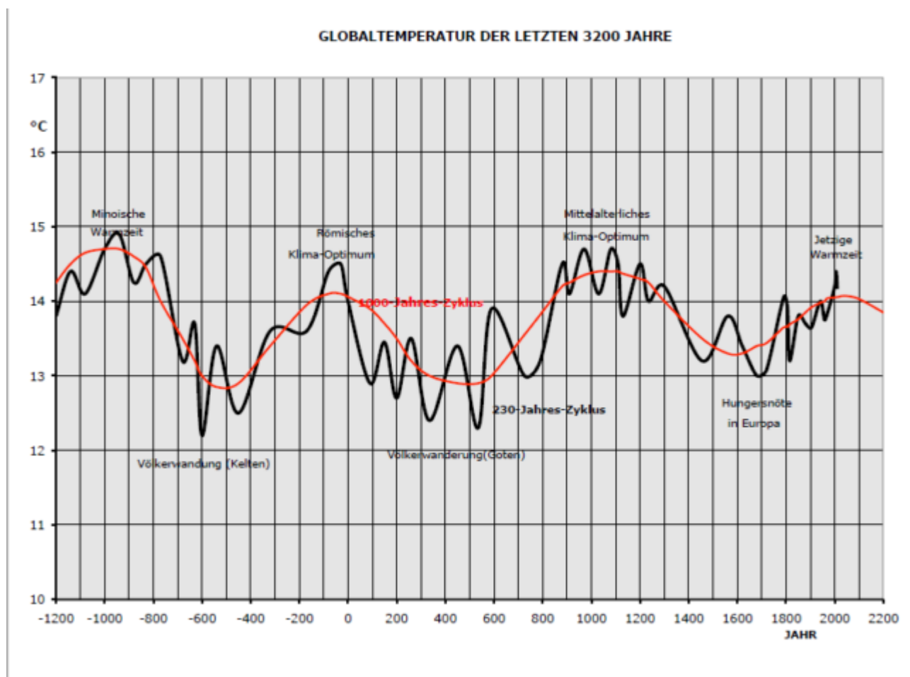
Bild 2: Der globale Temperaturwandel der letzten 3200 Jahre: die
