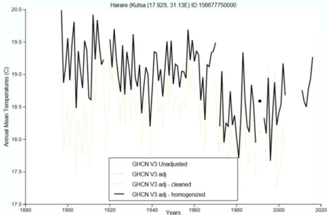
Bild 4.2 Temperaturverlauf Harare (Simbabwe) seit ca. 1900. Quelle: NASA
