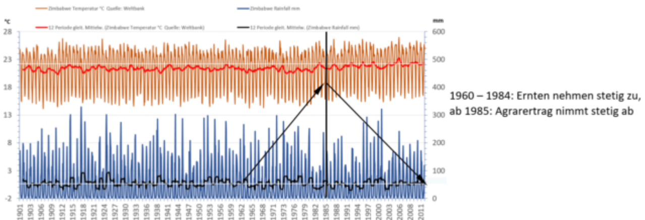
Bild 4 Simbabwe Temperatur (braun) und Niederschlag (blau) von 1901 – 2012 Quelle: THE WORLD BANK GROUP Climate Change Knowledge Porta. Zugefügt ist schematisch der Ernte-Ertragsverlauf von Bild 3 und 5
